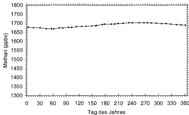
Abbildung 7.15 Methan Jahresgang an der Neumayer-Station 1997
