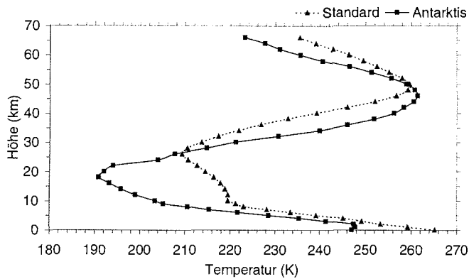
Abbildung 5.1 Temperaturprofil für Antarktis- und Standardbedingungen
