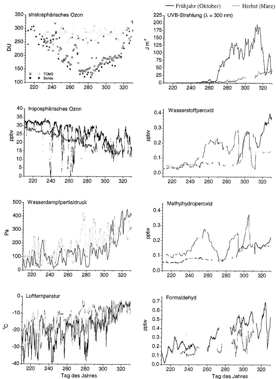
Abbildung 8.4 Vergleich für verschiedene Parameter zwischen Frühjahr und Herbst. Schwarz dargestellt sind die tatsächlichen Verhältnisse im antarktischen Frühjahr (Ozonloch). Grau dargestellt sind die im antarktischen Herbst beobachteten Mischungsverhältnisse. Diese wurden durch Spiegelung an einer gedachten Linie in der Mitte der Polarnacht so dargestellt, dass die Zeiten gleicher Sonnenstände übereinander zu liegen kommen.
