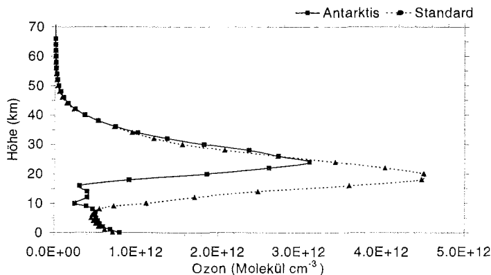
Abbildung 5.2 Ozonprofil für Antarktis- und Standardbedingungen
