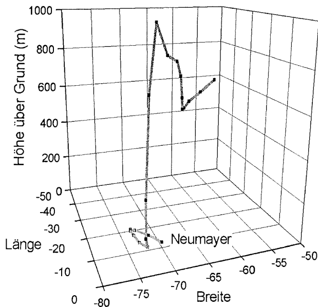
Abbildung 7.7 Vertikal-Komponente der bodennahen Trajektorie vom 26.06.97
