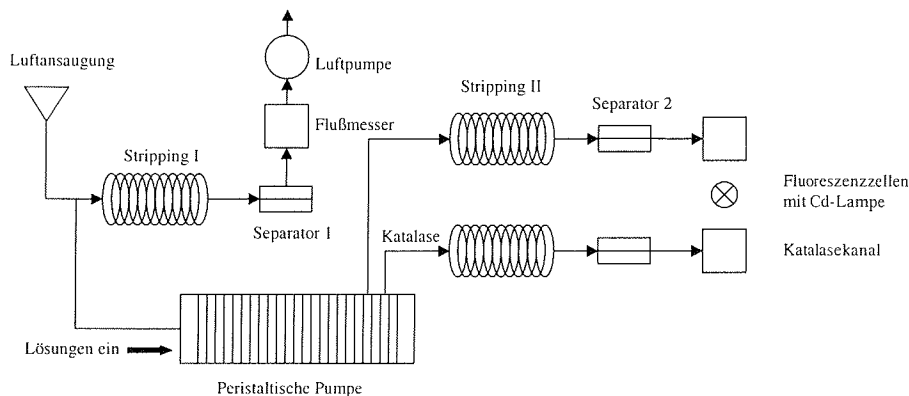
Abbildung 4.4 Schematische Darstellung des Peroxid Analysators
