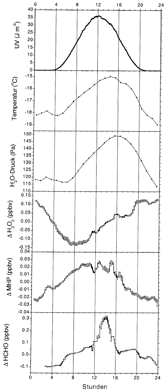
Abbildung 8.9 Tagesgänge verschiedener Größen: UV-Strahlung, Lufttemperatur, Wasserdampfpartialdruck, Differenz Wasserstoffperoxid, Differenz Methylhydroperoxid und Differenz Formaldehyd
