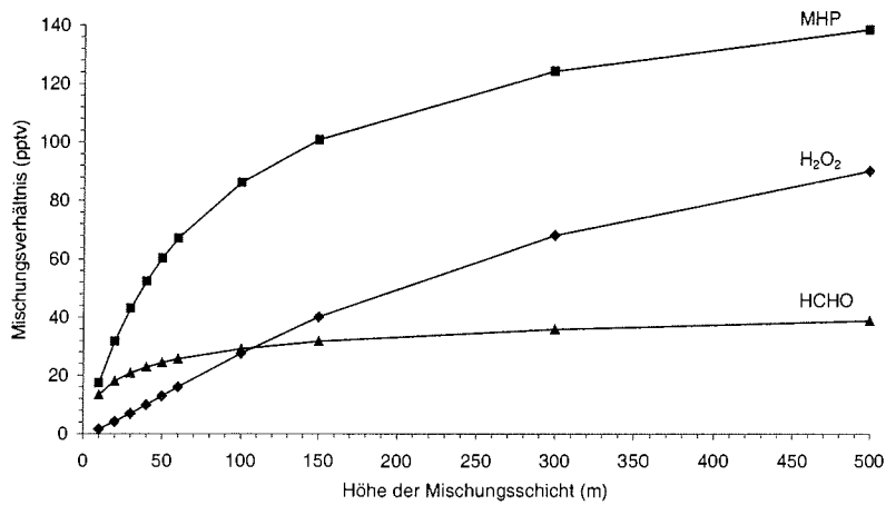
Abbildung 7.2 Einfluss der Grenzschichthöhe auf die Depositionsrates. Dargestellt sind die modellierten Mischungsverhältnisse von Wasserstoffperoxid, Methylhydroperoxid und Formaldehyd in Abhängigkeit von der Höhe der Mischungsschicht.
