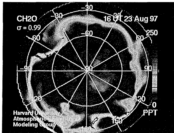
Abbildung 7.14 Modellerte bodennahe HCHO-Mischungsverhältnisse am 23. 08.97
