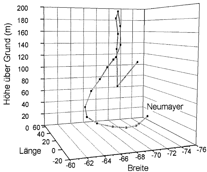
Abbildung 7.6 Vertikal-Komponente der bodennahen Trajektorie vom 25.06.97
