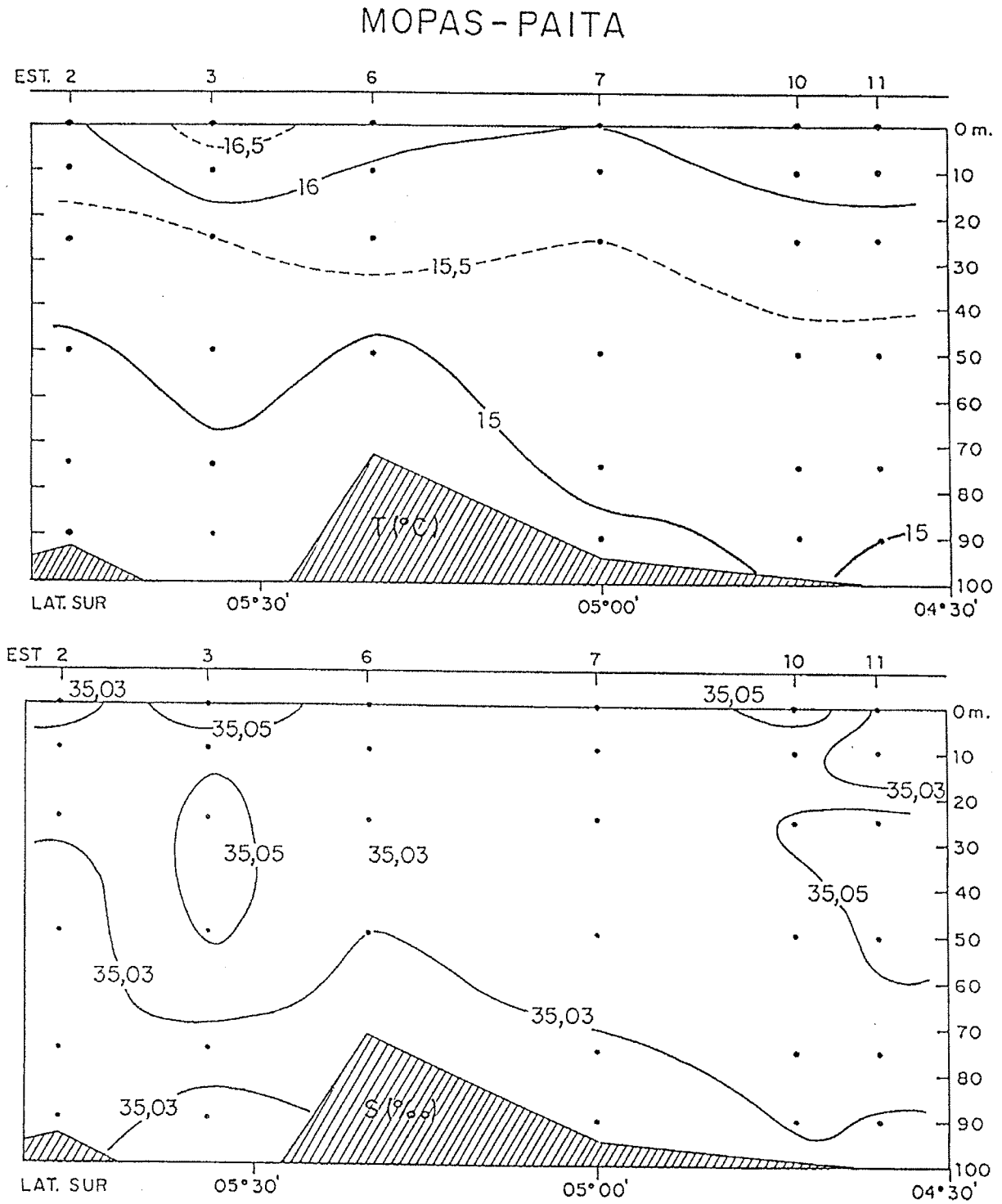
Fig. 4 Secciones Verticales Paralelas a la Costa de Temperatura y Salinidad, aproximadamente a 15 mn. MOPAS Paíta (20-22/08/95)
