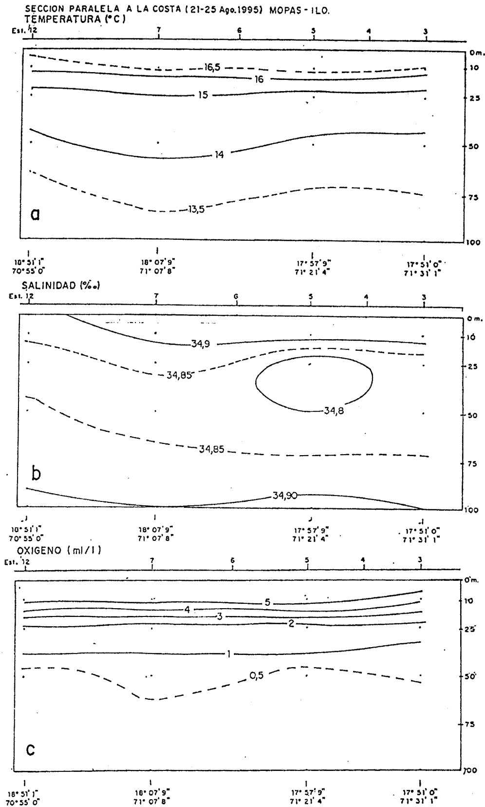
Fig.5 Secciones Verticales de Temperatura, Salinidad y Oxígeno, alrededor de los 15 mn frente a Ilo. Con Datos del MOPAS Ilo (21-25 Ago.1995).
