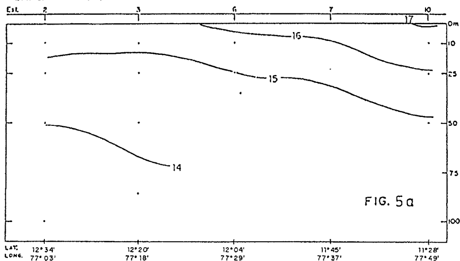
SECCION PARALELA A LA COSTA (15-18 Ago. 1995) MOPAS-CALLAO. SALINIDAD (‰)
