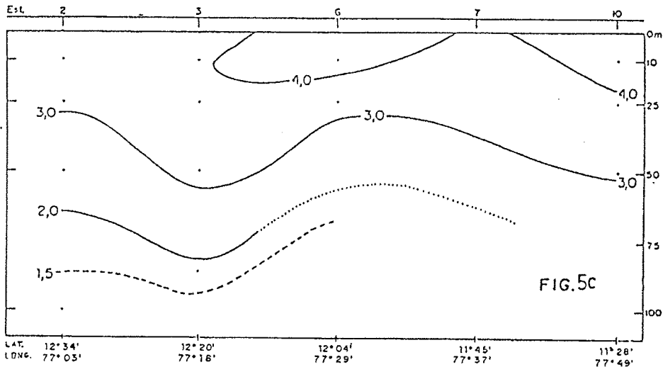
SECCION PARALELA A LA COSTA (15-18 Ago. 1995) MOPAS-CALLAO. OXIGENO (ml/l)
