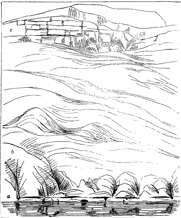
Ritenbenk's Kohlenbruch. a. Kohlenlager. b. Gelblicher Sandstein. c. Basalt.
