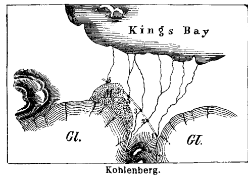
Steinkohlenlager der Kingsbai.
