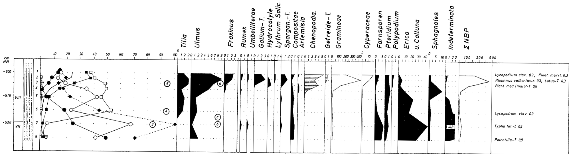
Abb. 6: Profil Gotteskoog-I (G-I) – Basistorf.
