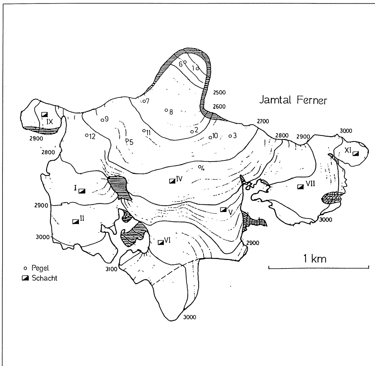
Abbildung 4: Lage der Schneeschnähte (Quadrate) und Pegel (Punkte) am Jamtal Ferner im April 1998. Die Meßergebnisse sind in Tabelle 3 zusammengefaßt.
