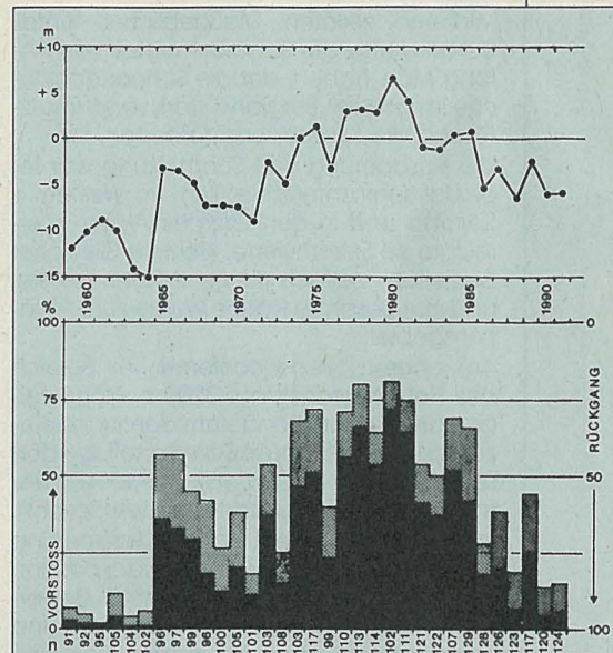
Diagramm 1: Die mittlere Längenänderung der Ostalpengletscher (oben) und die Anteile vorstoßender (schwarz), stationärer (punktiert) und zurückschmelzender (weiß) Gletscherenden von der Anzahl (n) der beobachteten Gletscher.
