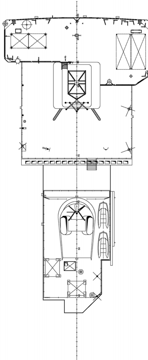
5. Aufbaudeck PEILDECK
