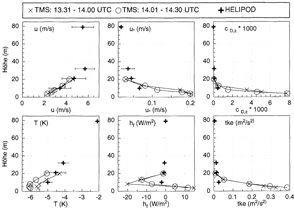
Abbildung 3.16: Vergleichsmessung von Helipod und TMS vom 18. August 1996.
