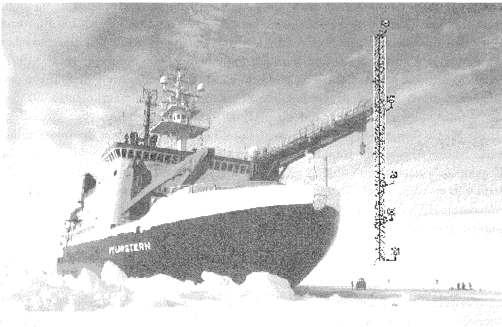
Abbildung 3.1: Ansicht von Polarstern während einer Messung. Die Anlage am Bugkran wurde grafisch hervorgehoben. Foto: C. Lüpkes
