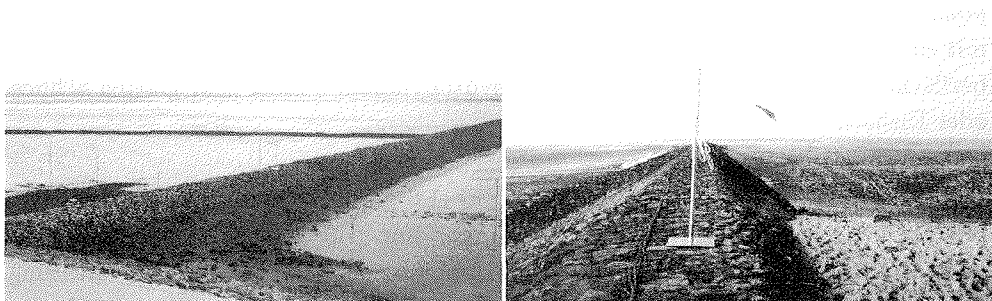
Abbildung 3.10: Ansicht der Buhnen, an denen Strömungsmessungen vorgenommen wurden. Die Buhnenhöhen betragen 1.6 m (links) und 2.6 m (rechts).
