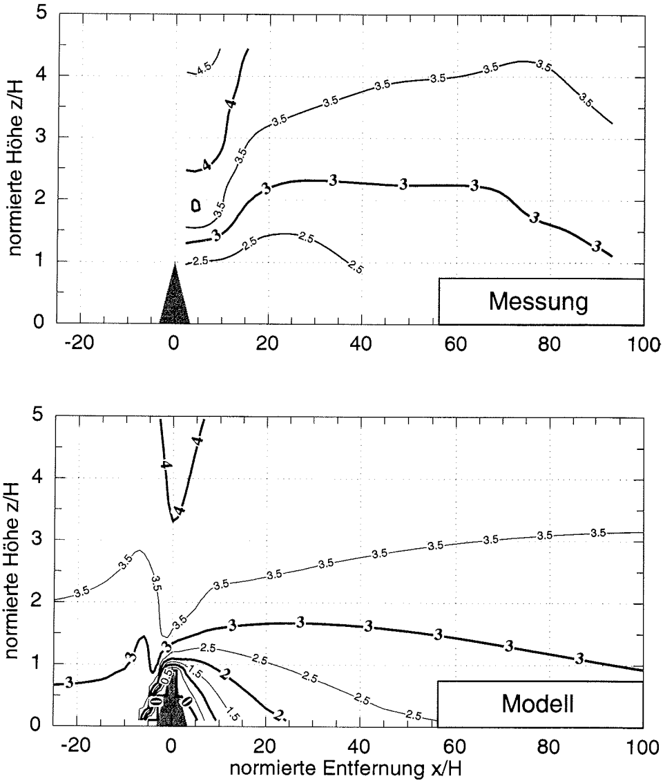
Abbildung 5.12: Ein Vergleich der horizontalen Windgeschwindigkeit bei Naturmessung (oben) und Modellrechnung (unten) nach Lopez (2001). Höhen- und Abstandsangaben sind mit der jeweiligen Hindernishöhe normiert.
