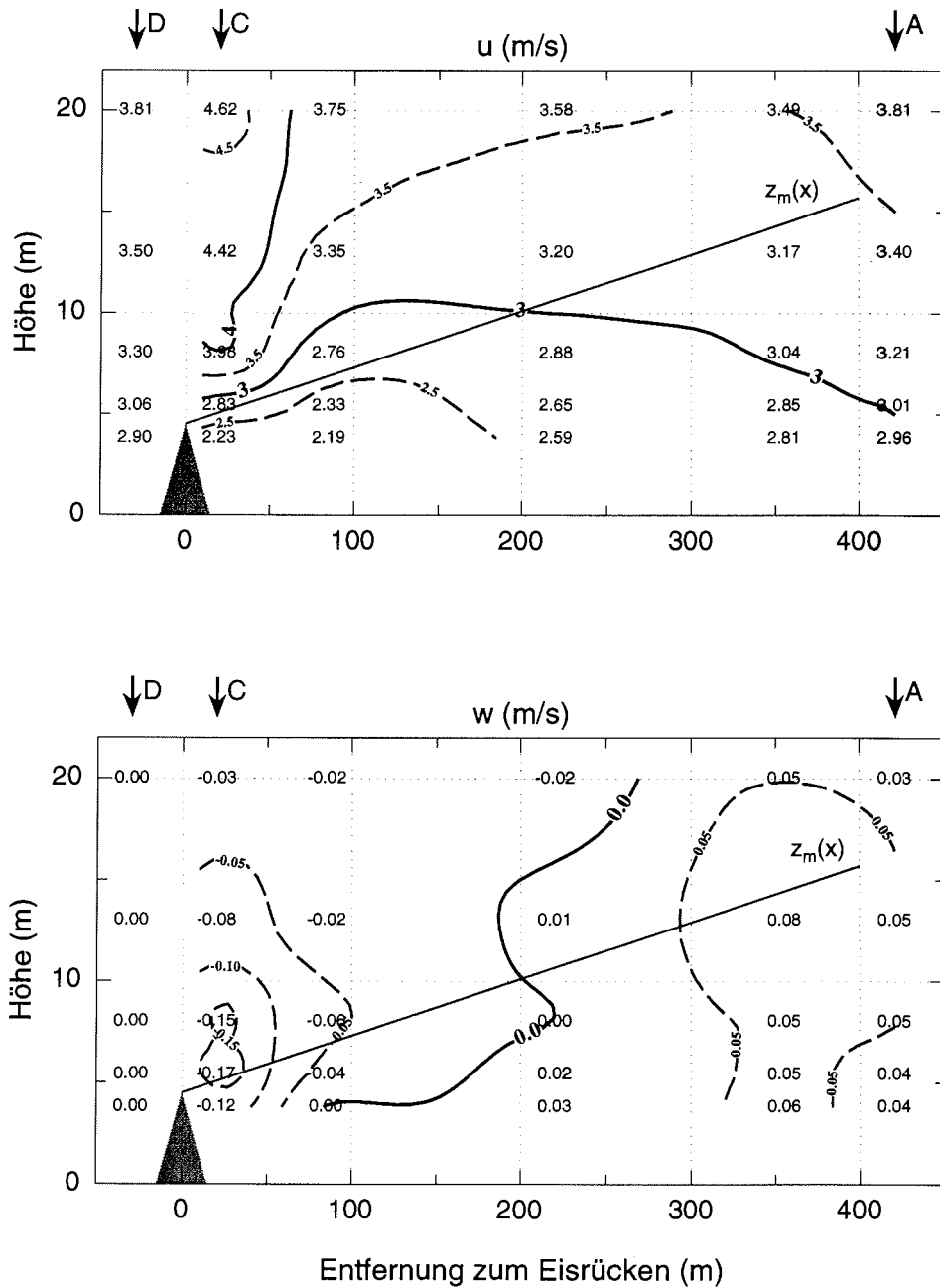
Abbildung 5.4: Isolinien von u (oben) und w (unten) am 13. August 1996. Die Positionen der stationären Messungen sind am oberen Rand durch Pfeile markiert. Die Gerade markiert den Anstieg des Turbulenzmaximums gemäß der Gleichung (5.1).
