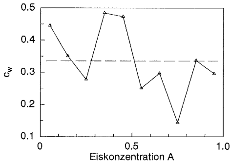
c_w = 0.335 Abbildung 5.11: Der Widerstandsbeiwert c_w von Eisschollen, als Funktion der Eiskonzentration.
