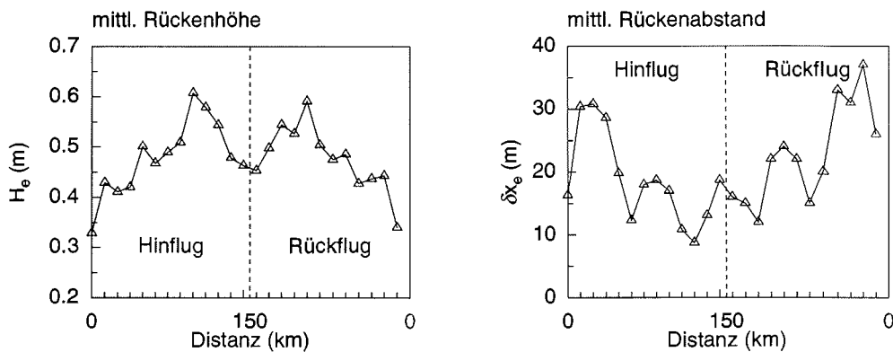
Abbildung 3.9: Mittelwerte von Eisrückenhöhe (links) und -abstand (rechts) während des ARTIST-Meßfluges am 16. März 1998.
