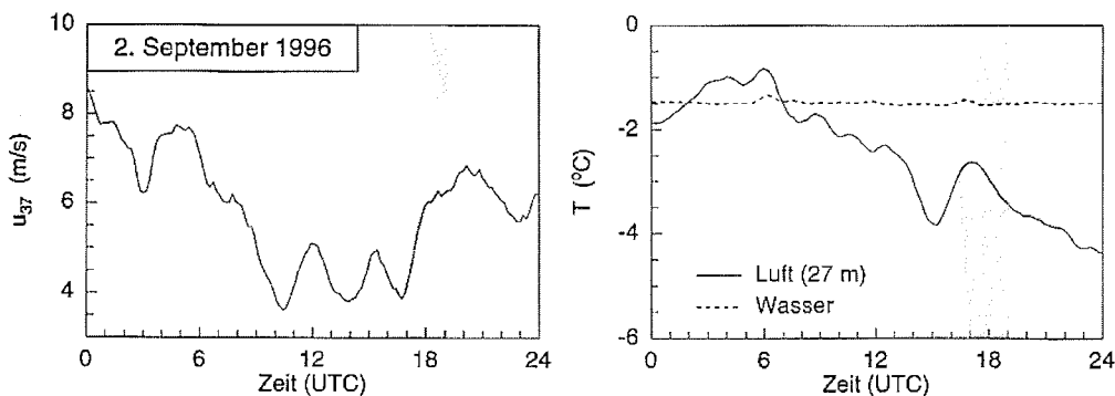
Abbildung 4.2: Zeitlicher Verlauf von u_{37} sowie der Temperaturen von Luft und Wasser am 2. September 1996, basierend auf Messungen des PODEV-Systems. Der Zeitraum des Polynja-Experimentes ist grau unterlegt.
