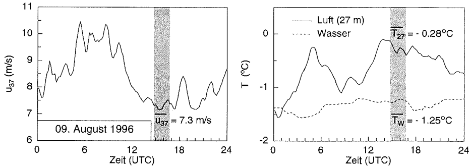
Abbildung 4.7: Zeitreihen von u_{37} , T_{27} und T_W am 9. August 1996 (PODEV-System). Grau unterlegt ist der Zeitraum des Polynja-Experimentes.
