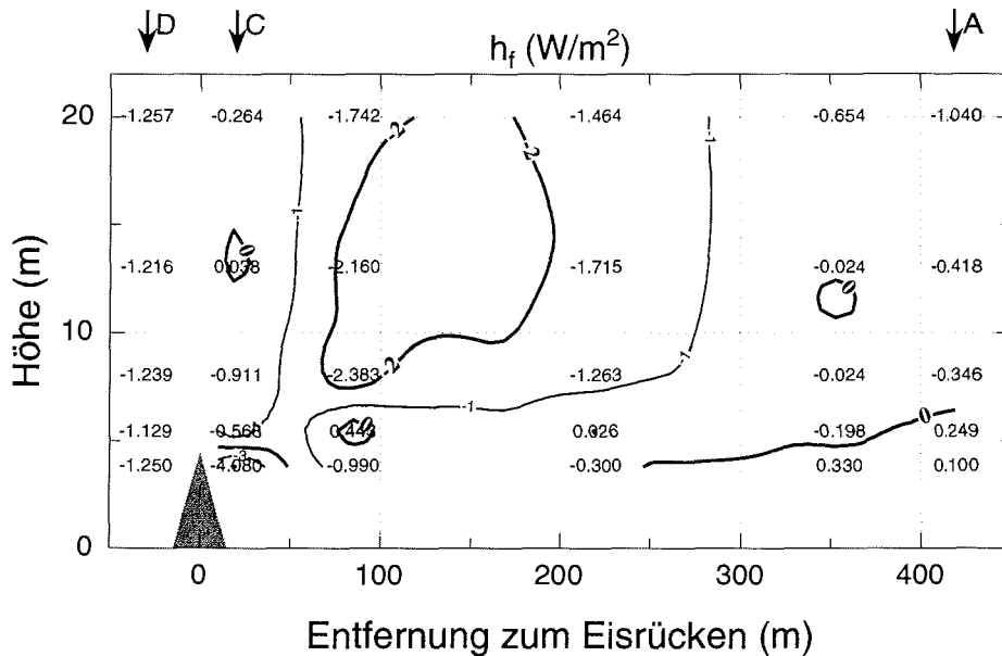
Abbildung 5.6: Isolinien des turbulenten Wärmeflusses h_f am 13. August 1996.
