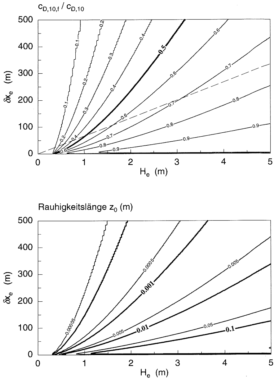
Abbildung 6.6: Der Quotient c_{D,10,f}/c_{D,10} (oben) bei neutraler Schichtung und die Rauigkeitslänge z_0 (unten) als Funktion von H_e und \delta x_e . Gestrichelte Linie: Ensembleaspektverhältnis A_e = H_e/\delta x_e = 0.015 .
