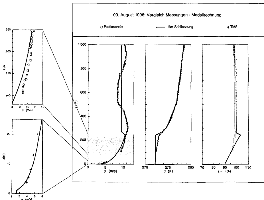
Abbildung 4.11: Vergleich der Meßwerte von u , \Theta und r.F mit dem Ergebnis der 1D-Studie. Für u sind die Überschneidungsbereiche zwischen den Messungen und der Modellrechnung vergrößert dargestellt.
