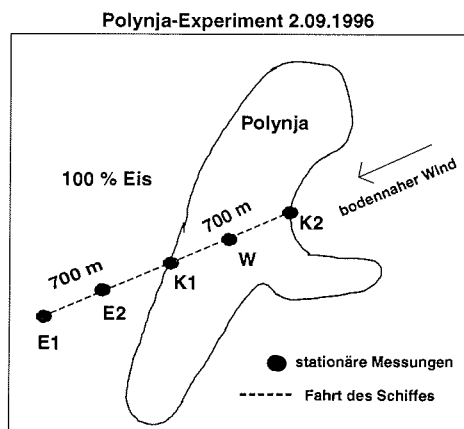
Abbildung 4.1: Das Polynjaexperiment am 2.09.1996. Die gestrichelte Linie kennzeichnet die Fahrt von Polarstern entgegen der mittleren Windrichtung (siehe Pfeil). Stationäre Messungen sind mit Punkten und den im Text verwendeten Stationenkennungen markiert.
