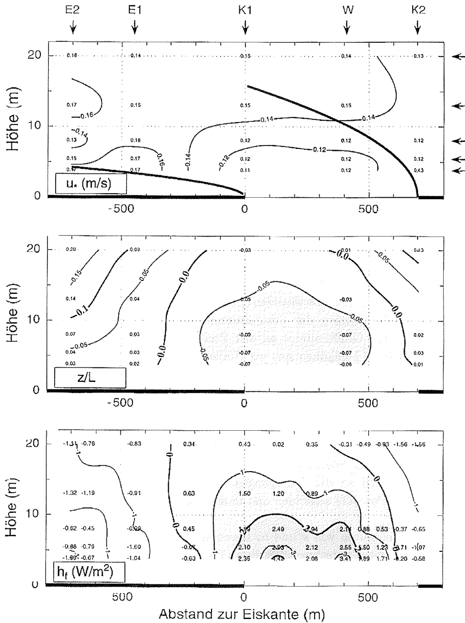
Abbildung 4.4: Isolinien­darstellung von u_* (oben), z/L (Mitte) und h_f (unten) am 2. September 1996. Die Obergrenze der internen Grenzschichten ist durch Linien angedeutet. Der Bereich der Meereisbedeckung ist durch schwarze Balken am unteren Rand gekennzeichnet, die stationären Meßpositionen sind am oberen Rand markiert. Die Anströmung erfolgte von rechts (Pfeile).
