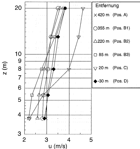
Abbildung 5.3: Die Vertikalprofile von u am 13. August 1996, in Abhängigkeit vom Abstand zum Eisrücken.
