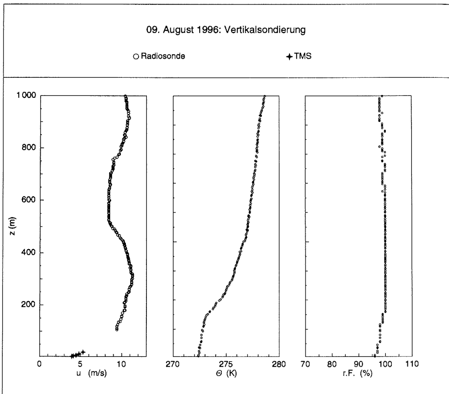
Abbildung 4.6: Radiosondenmessung vom 9. August 1996, 16 Uhr. Dargestellt sind die Windgeschwindigkeit u , die potentielle Temperatur \Theta und die relative Feuchte r.F. Bei u sind zusätzlich die TMS-Messungen (Rauten) eingezeichnet.
