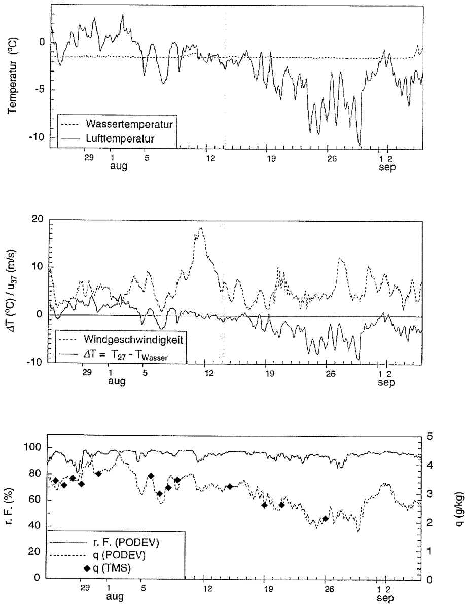
Abbildung 3.6: Luft- und Wassertemperatur (oben), Temperaturdifferenz \Delta T = T_L - T_W und Windgeschwindigkeit (Mitte), sowie spezifische Feuchte q und relative Feuchte r.F. (unten) während ARK XII. Die grau unterlegte Fläche markiert fehlende Daten der Wassertemperatur.
