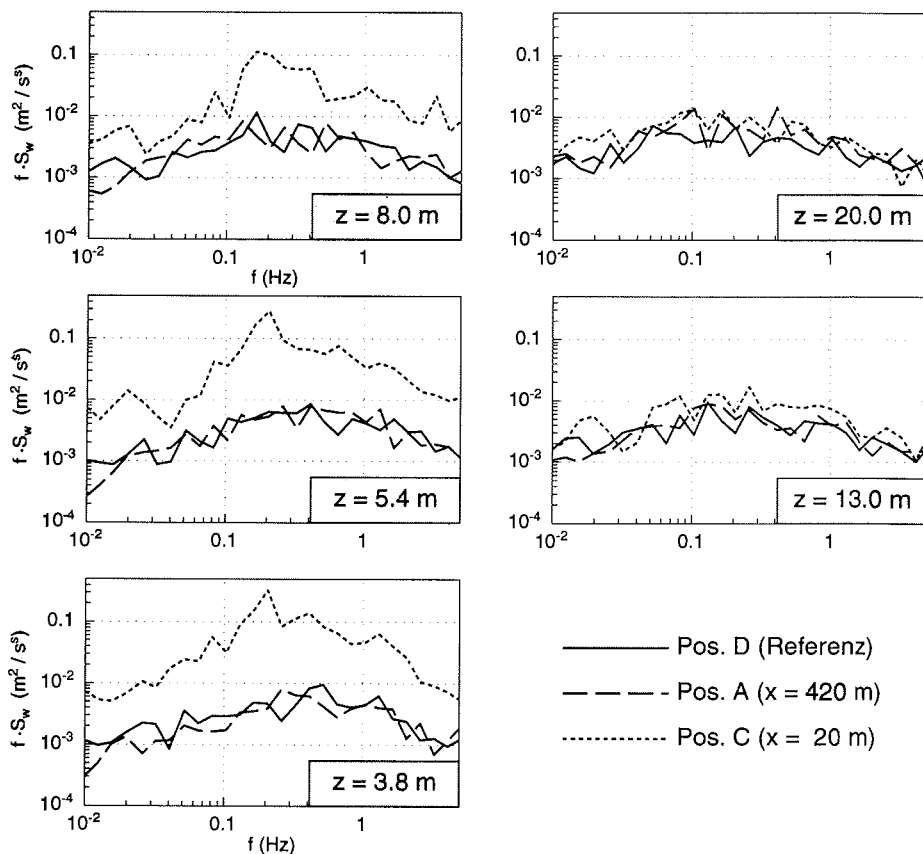
Abbildung 5.7: Varianzspektren der Vertikalkomponenten der Windgeschwindigkeit am 13. August 1996 für alle fünf Meßhöhen an den Positionen A, C und D.
