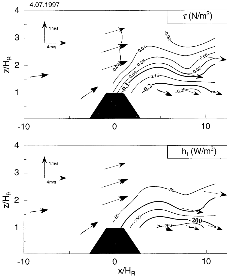
Abbildung 5.15: Isolinien von \tau (oben) und h_f (unten) am 4. Juli 1997. Unterlegt sind Windpfeile, entsprechend der Skala am linken oberen Rand. Höhen- und Abstandsangaben sind mit H_R = 1.6 \text{ m} normiert.
