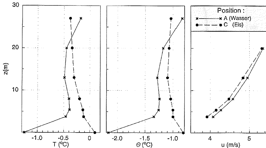
Abbildung 4.8: Vertikalprofile der Temperatur (links), der potentiellen Temperatur (Mitte) und der Windgeschwindigkeit (rechts) in der oberflächennahen Luftschicht, gemessen über Wasser (durchgezogen) und über Eis (gestrichelt).
