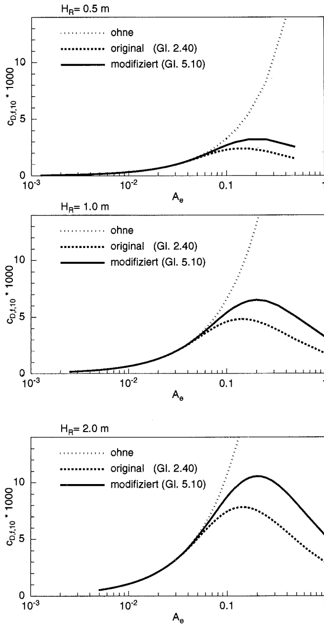
Abbildung 6.5: Der Formwiderstandskoeffizient c_{D,10,f} als Funktion des Ensembleaspektverhältnisses bei drei verschiedenen Rückenhöhen. Der Abschattungseffekt wurde vernachlässigt (Punkte) sowie durch die original (gestrichelt) und die modifizierte (durchgezogen) Nägeli-Formel gerechnet.
