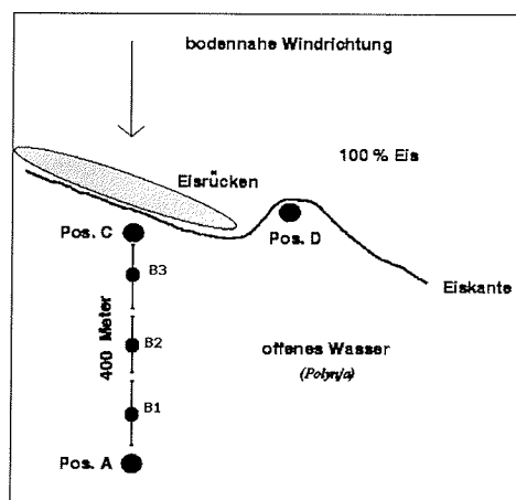
Abbildung 5.1: Prinzipskizze des Eisrückenexperimentes am 13. August 1996. Die Positionen stationärer Messungen sind durch Punkte markiert.
