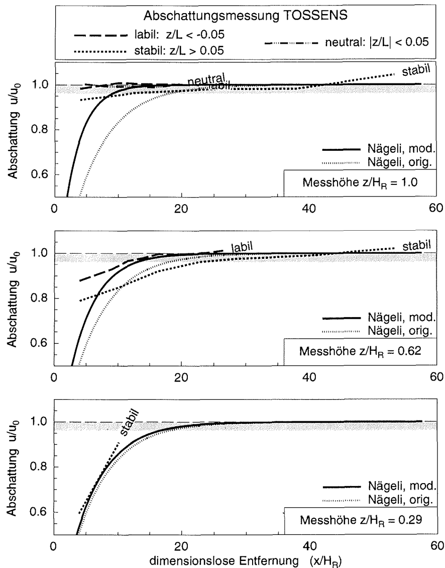
Abbildung 5.14: Die Abschattung u(z)/u_0(z) im Lee der Bühne mit H_R = 2.6 m in den Meßhöhen z/H_R = 0.29 (unten), 0.62 (Mitte) und 1.0 (oben) sowie bei unterschiedlicher atmosphärischer Schichtung. Ferner ist Gleichung (2.40) eingezeichnet. Die Entfernungs- und Höhenangaben sind mit der Bühnenhöhe H_R = 2.6 m normiert. Der grau schraffierte Bereich symbolisiert eine Abweichung um \pm 3.8\% des Anströmwertes.
