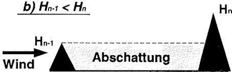
Abbildung 6.1: Schema zur Fallunterscheidung des Abschattungseffektes bei dicht stehenden Rücken ( A > 0.015 ). Im oberen Fall wirkt die Abschattung auf den gesamten folgenden Rücken, während im unteren Fall lediglich ein Teilbereich des nächsten Eisrückens betroffen ist.
