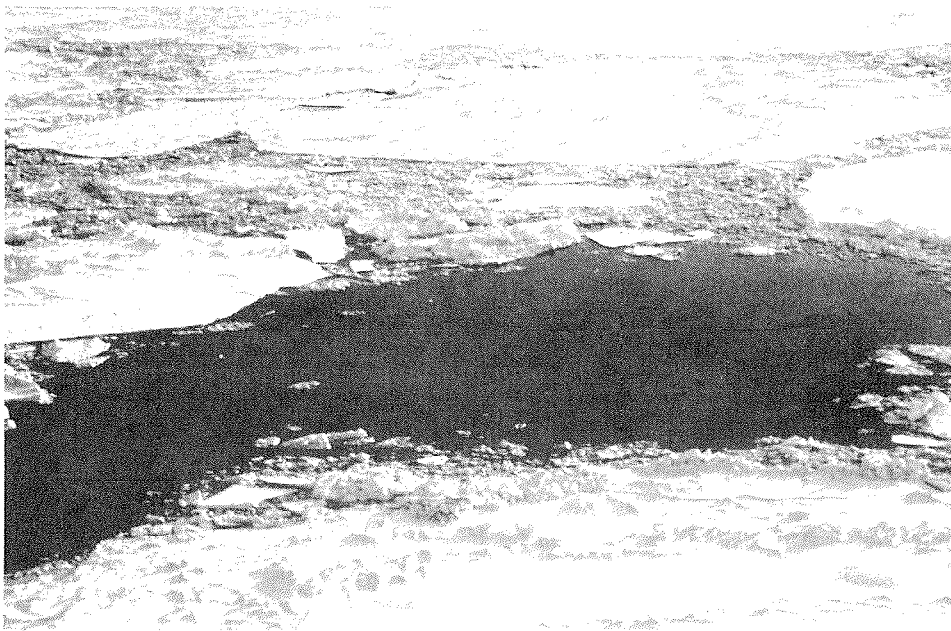
Abbildung 1.1: Ausschnitt der arktischen Eisrandzone im Frühjahr, aufgenommen im April 1998 vor der Südküste Spitzbergens (bei einer Flughöhe von etwa 30 Metern).
