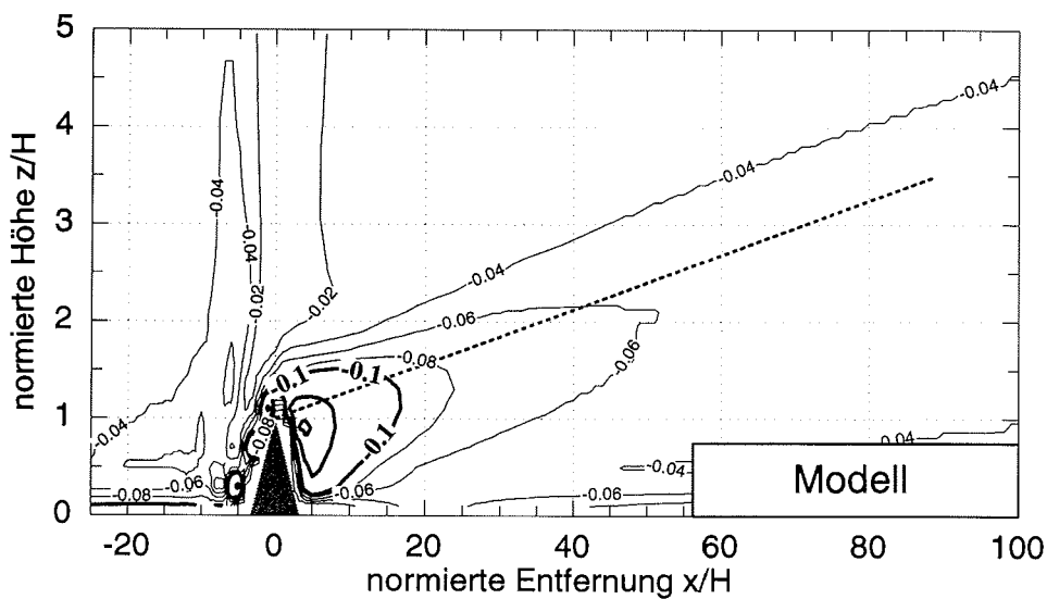
Abbildung 5.13: Ein Vergleich des Impulsflusses bei Naturmessung (oben) und Modellrechnungen (unten) nach Lopez (2001). Höhen- und Abstandsangaben sind mit der jeweiligen Hindernishöhe normiert. Zusätzlich ist der Anstieg des maximalen Impulsflusses nach Gleichung (5.1) mit \bar{a} = 0.028 eingezeichnet (gestrichelte Linie).
