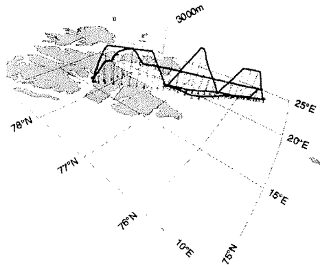
Abbildung 3.7: Flugweg der Polar-2-Mission am 16. März 1998 im Eingangsbereich des Storefjordes, südöstlich von Spitzbergen (aus Hartmann et al., 1999).
