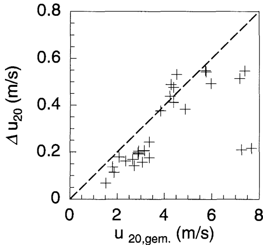
Abbildung 3.14: Die Differenz \Delta u_{20} = u_{20,\text{gem.}} - u_{20,\text{extrap.}} als Funktion von u_{20,\text{gem.}} . Die gestrichelte Gerade entspricht einer Abweichung vom Meßwert u_{20,\text{gem.}} um 10 %.
