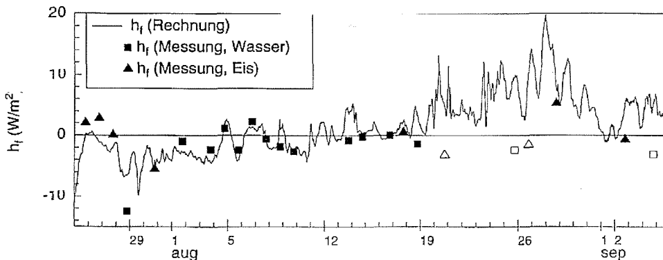
Abbildung 4.13: Abgeschätzter (Linie) und gemessener (Symbole) Wärmefluß der ARK XII-Kampagne. Während des grau unterlegten Zeitraumes sind keine Daten der Wassertemperatur verfügbar. Quadrate: über Wasser, Dreiecke: über Eis, offene Symbole: schlechte Übereinstimmung zwischen Meß- und Schätzwert.
