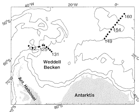
Abb. 16: Positionen der in dieser Arbeit verwendeten Stationen M11/5-Expedition (1990). Tiefenlinien sind 1000, 3000 und 5000 m.
