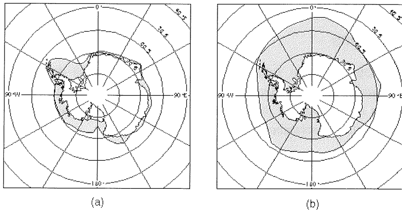
Abb. 3: Mittlere Meereisausdehnung des Südlichen Ozeans der Jahre 1973 – 1993 a) im Februar; b) im Oktober [Simmonds und Jacka, 1995]
