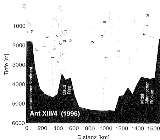
Abb. 22: Strömungsfeld des Null-Meridian-Schnitts aus mit Schiffs-ADCP angepassten CTD-Daten
