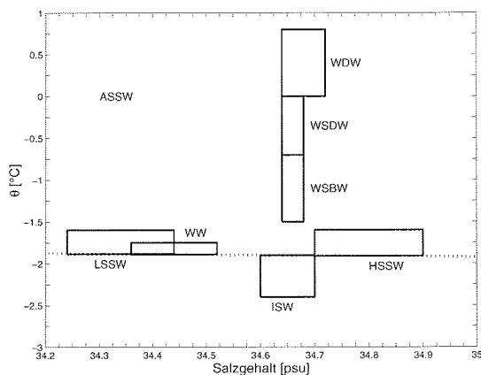
Abb. 5: Schematische Darstellung der Hauptwassermassen des Weddellmeeres im \theta -S-Raum, die gestrichelte Linie stellt den Oberflächen-Gefrierpunkt dar (nach [Foldvik et al., 1985c])
