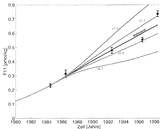
Abb. 34: Berechneter Verlauf der F11 Konzentration des südlichen Kerns. Die schwarze Linie ist mit der Referenz-Altersverteilung (in Kapitel 6.4 bestimmten) berechnet, für die grauen Linien wurden alle Anteile seit 1980 mit den angegebenen Faktoren versehen.
