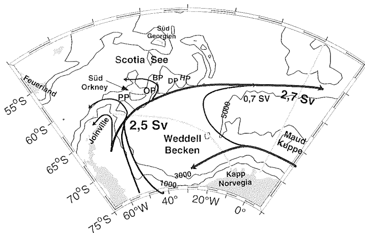
Abb. 36: Strömung des frisch belüfteten Wassers des nördlichen Kerns; graue Linien stellen die Schnitte dar, die Pfeile die Strömung des frisch belüfteten Wassers; PP = Philip-Passage, OP = Orkney-Passage, BP = Bruce-Passage, HP = Hoyer-Passage
