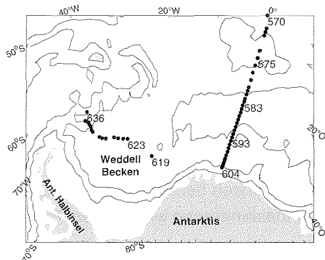
Abb. 17: Positionen der in dieser Arbeit verwendeten Stationen der ANT X/4-Expedition (1992). Tiefenlinien sind 1000, 3000 und 5000 m.
