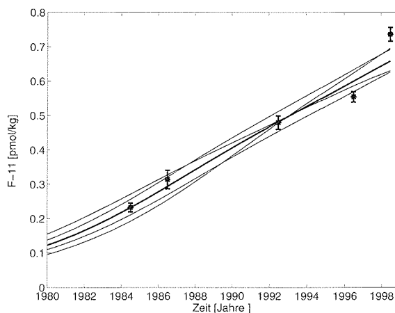
Abb. 31: Berechneter Verlauf der F11 Konzentration des südlichen Kerns. Die dicke Linie zeigt den Verlauf für die Parameter des Minimums bei \sigma = 4 Jahre, die dünneren den der Kreuze um das Minimum in Abb. 30. Außerdem sind die gemessenen mittleren Konzentrationen (und Fehler) des südlichen Kerns dargestellt (siehe Tabelle 19)
