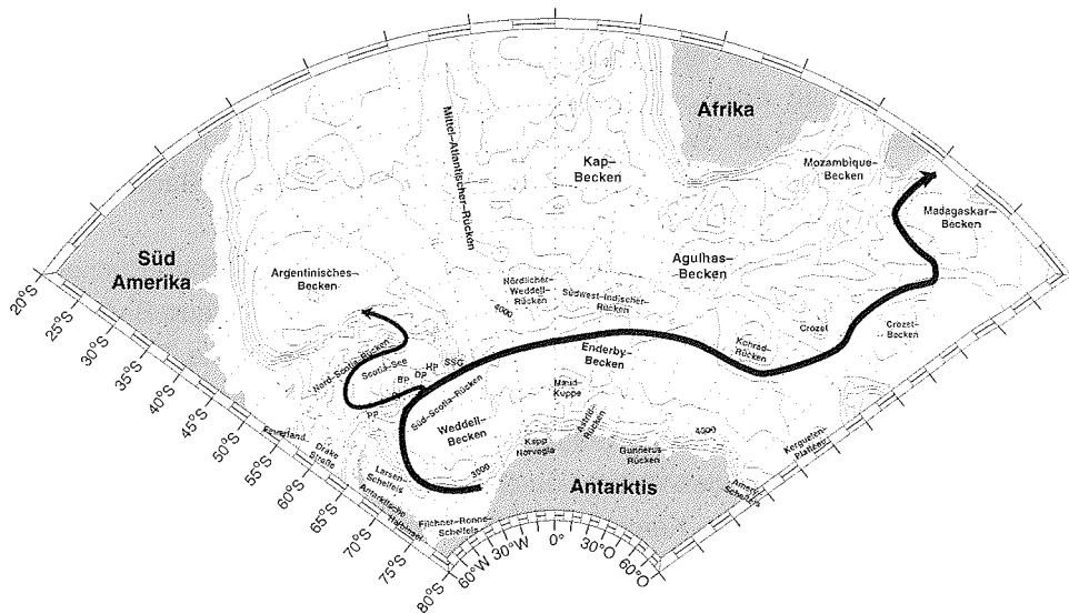
Abb. 7: Schematische Darstellung des Ausstroms von im Weddellmeer gebildeten Tiefen- und Bodenwassers in den Atlantischen und Indischen Ozean; nach [Locarnini et al., 1993; Haine et al., 1998]
