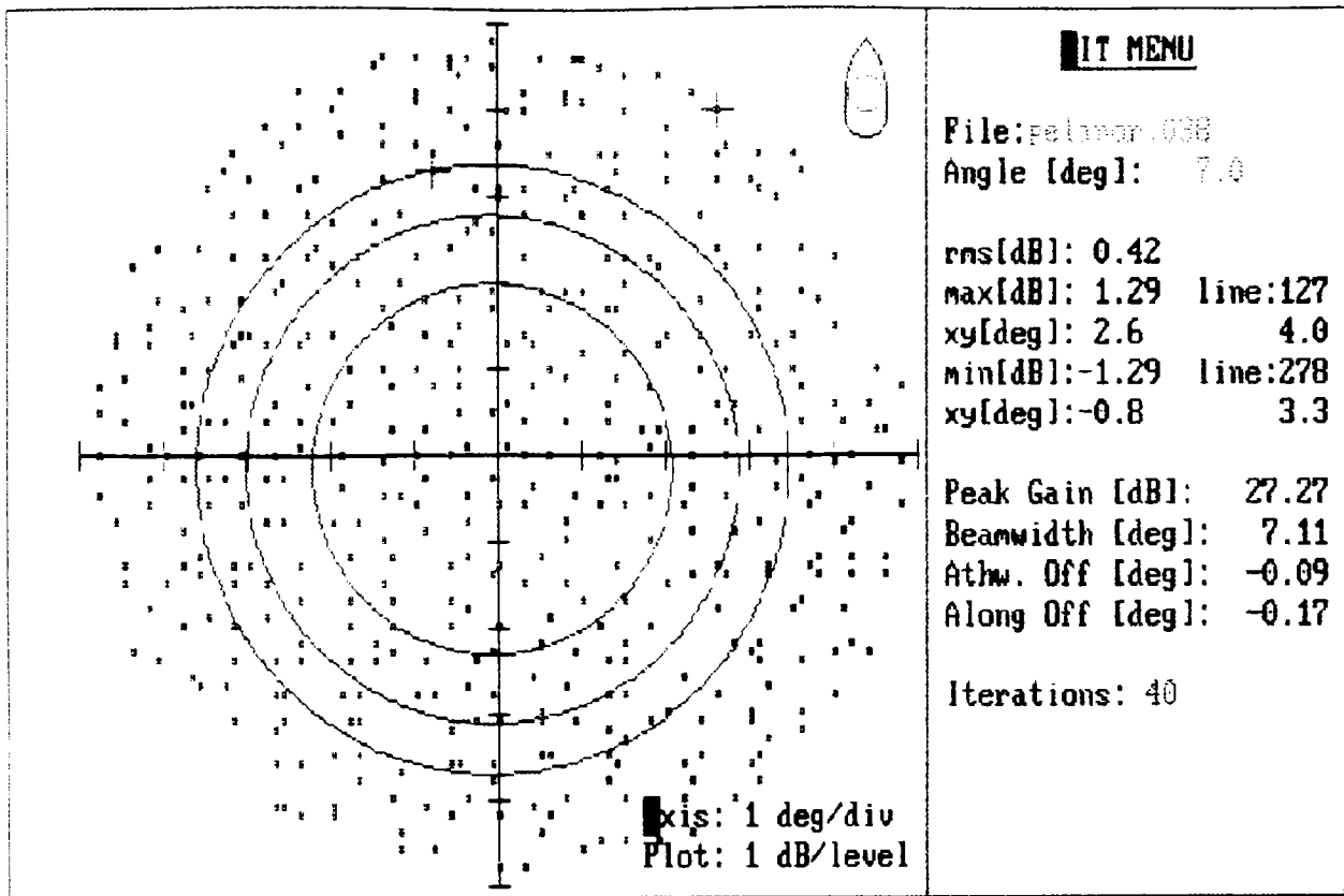
Figura 41. Patrón de directividad medido en la frecuencia de 38 KHz del B/I Carlos Porter. Crucero PELANOR 9308-09.
