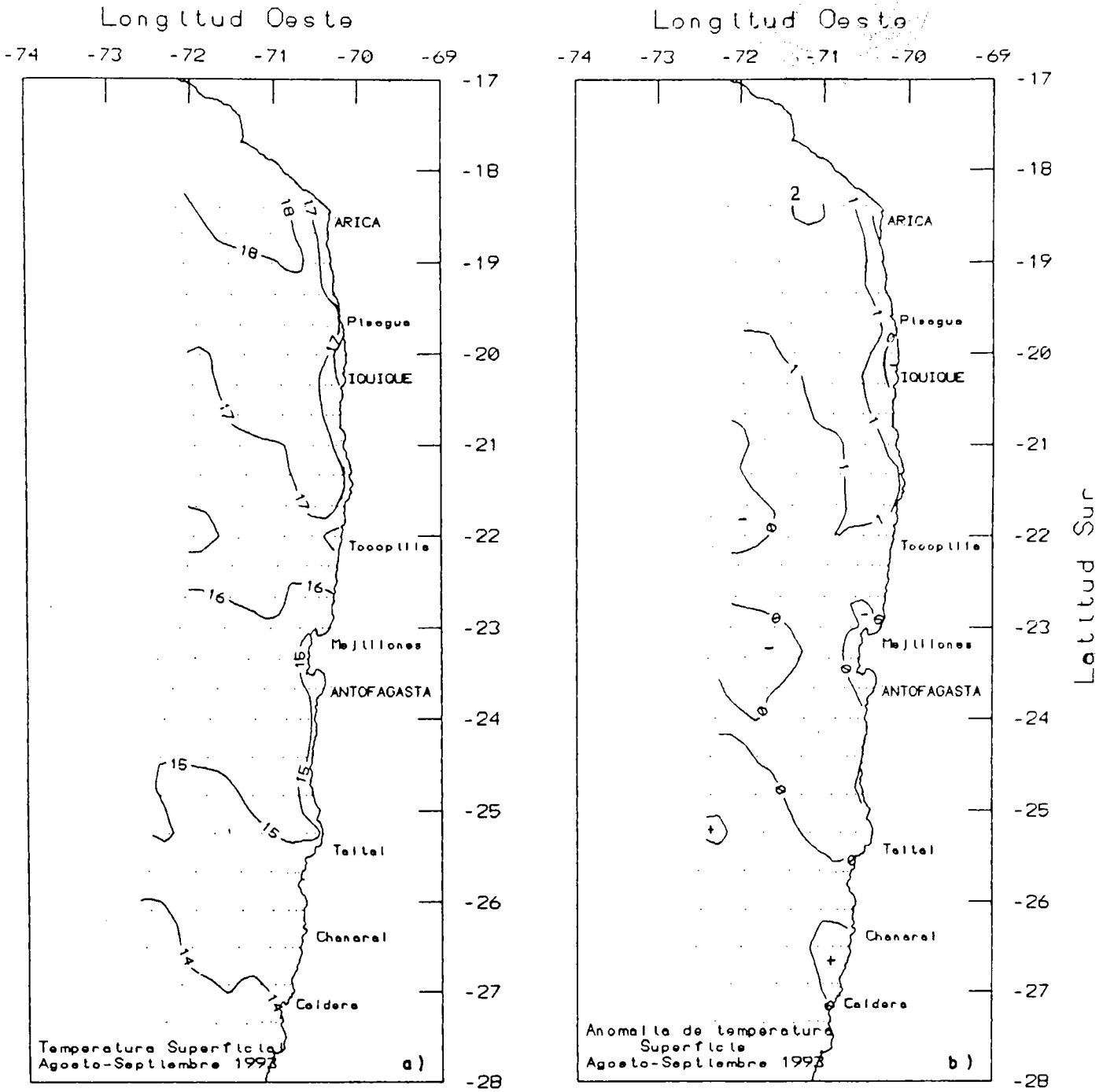
Figura 4. Distribución superficial de a) temperatura ( ^{\circ}\text{C} ) y b) anomalía de la temperatura ( ^{\circ}\text{C} ) respecto a los promedios de largo plazo de Reynolds. Agosto-Septiembre de 1993. CRUCERO PELANOR 9308-09.
