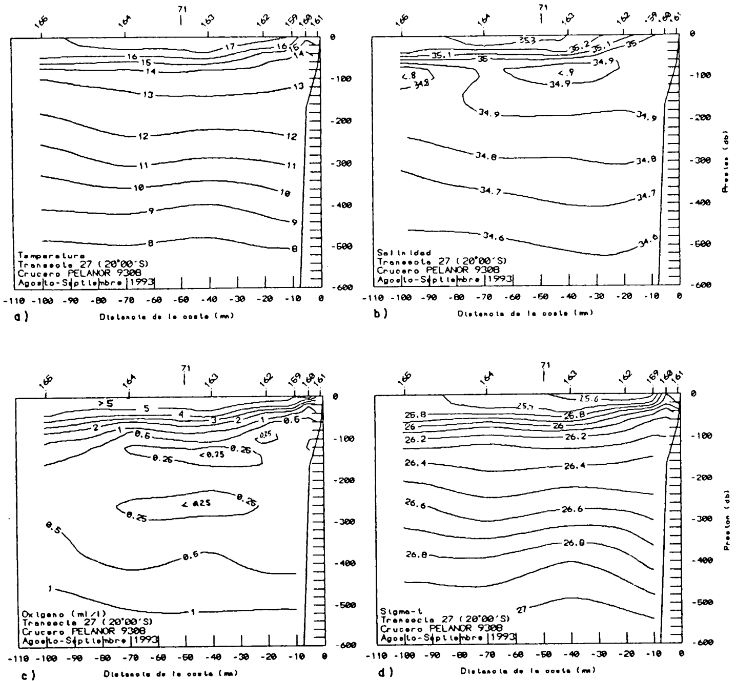
Figura 7. Distribución vertical de a) temperatura ( ^{\circ}\text{C} ), b) salinidad, c) concentración de oxígeno disuelto y d) densidad, en la transecta 27. Agosto-Septiembre de 1993. CRUCERO PELANOR 9308-09.
