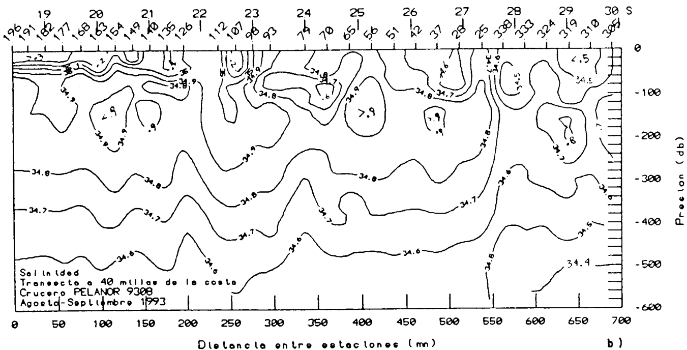
Figura 89. Distribución vertical de a) temperatura ( ^{\circ}\text{C} ), y b) salinidad, a lo largo de una transecta a 40 millas de la costa. Agosto-Septiembre de 1993. CRUCERO PELANOR 9308-09.
