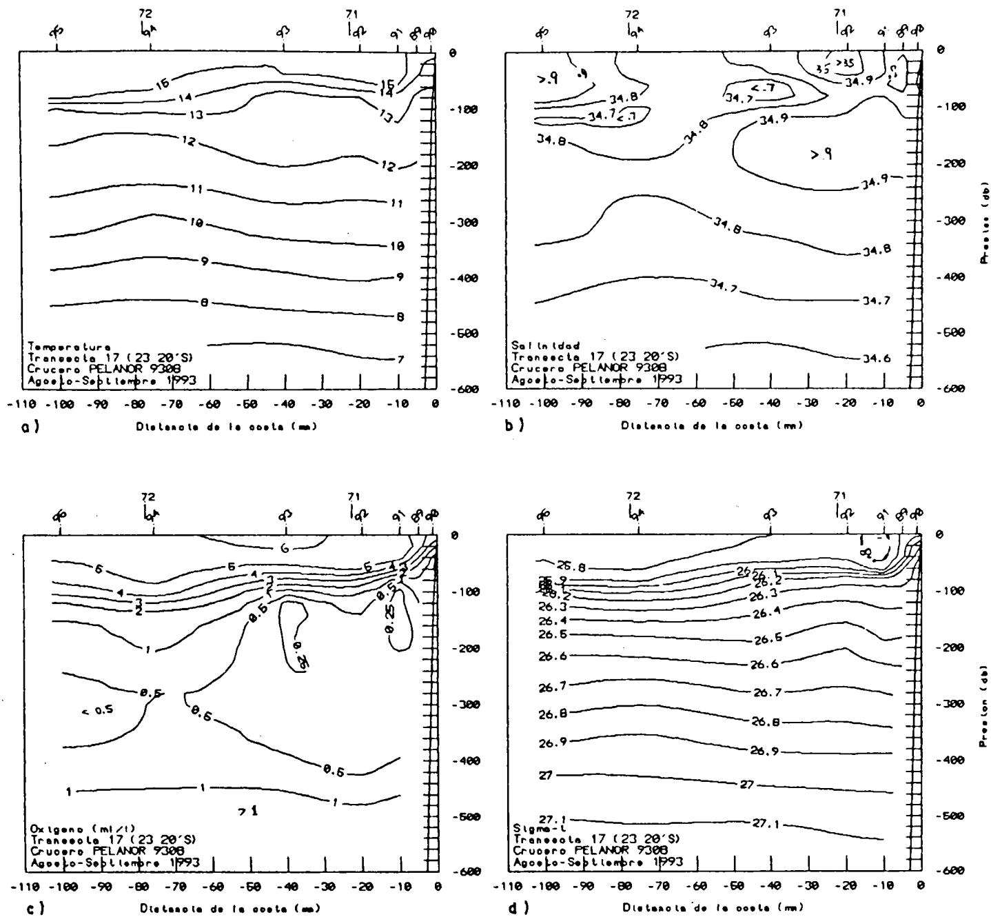
Figura 11. Distribución vertical de a) temperatura ( ^{\circ}\text{C} ), b) salinidad, (c) concentración de oxígeno disuelto y d) densidad, en la transecta 17. Agosto-Septiembre de 1993. CRUCEIRO PELANOR 9308-09.
