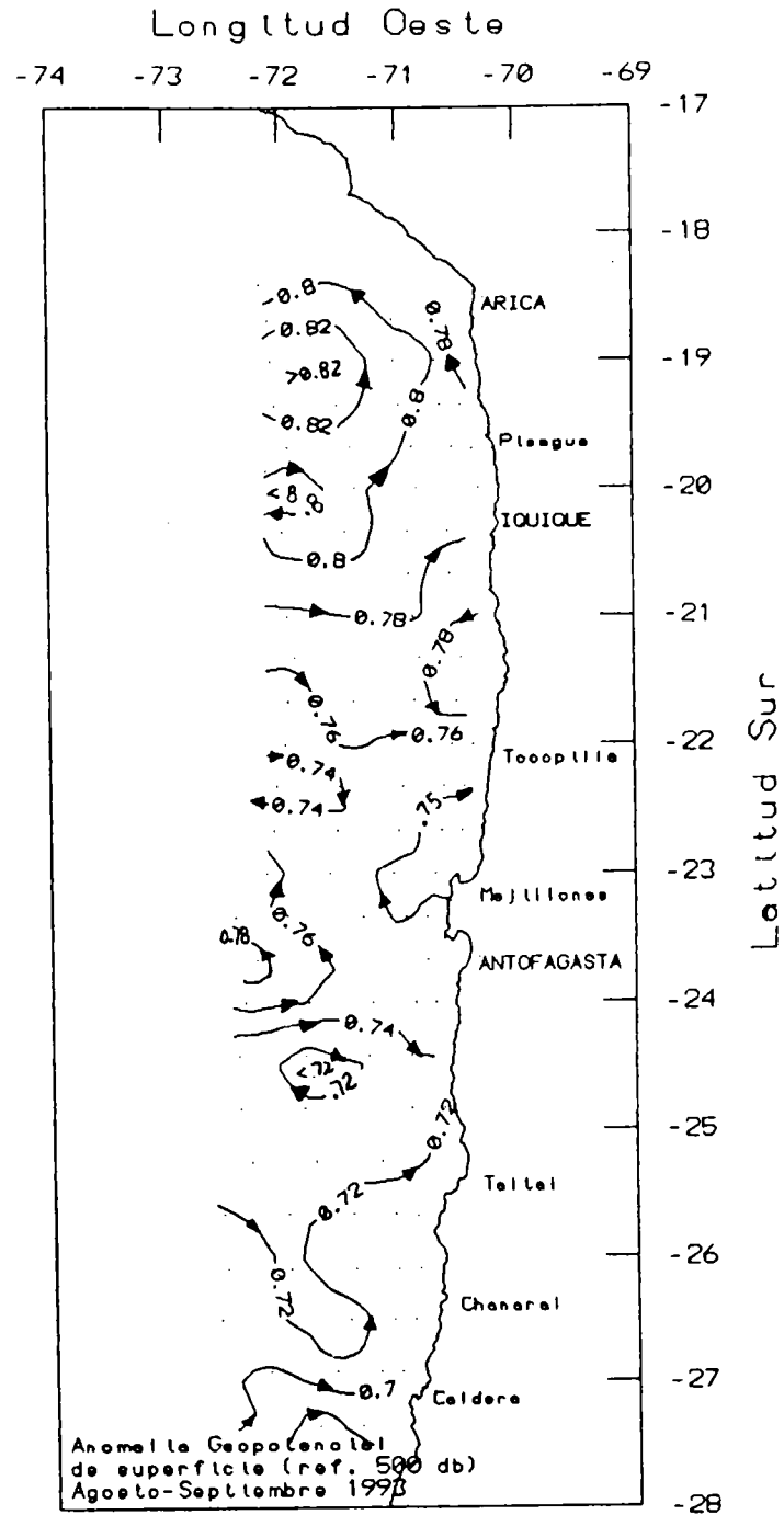
Figura 19. Distribución de la anomalía geopotencial de superficie referida a 500 db, durante Agosto-Septiembre de 1993. CRUCERO PELANOR 9308-09.
