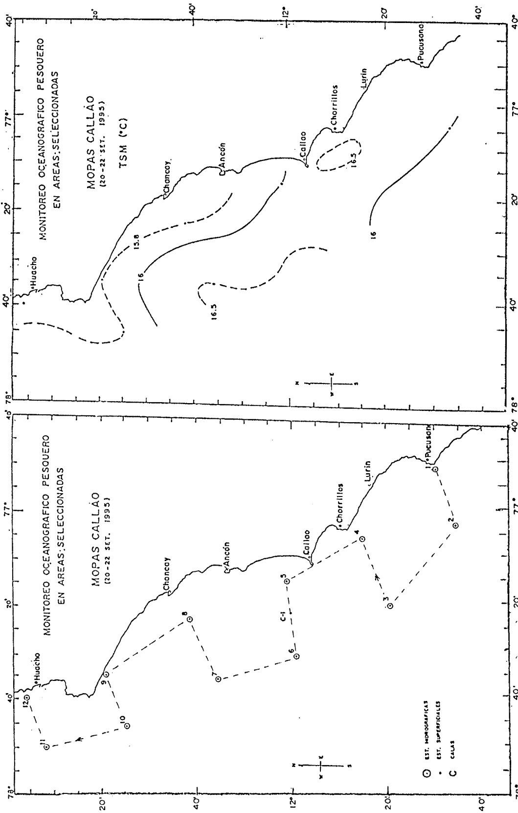
Fig. 9 Carta de trayectos y estaciones MOPAS Callao (20-22/09/95) Fig. 10 Distribución de la temperatura superficial del mar MOPAS Callao
