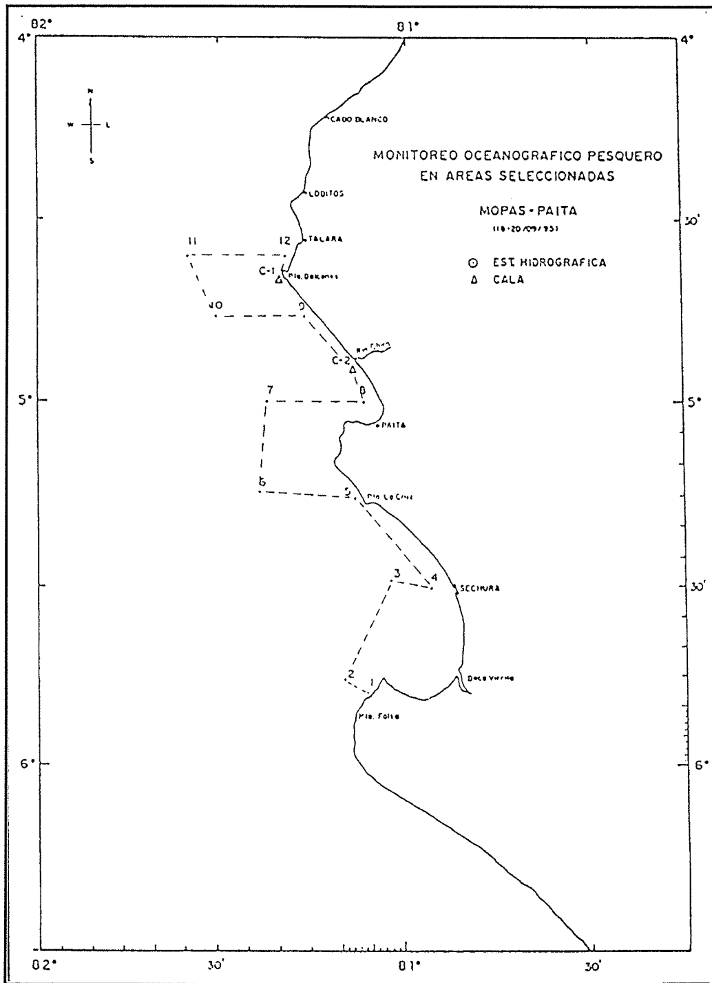
Fig. 1 Carta de trayecto y estaciones. MOPAS Paita (18-20/09/ 95)
