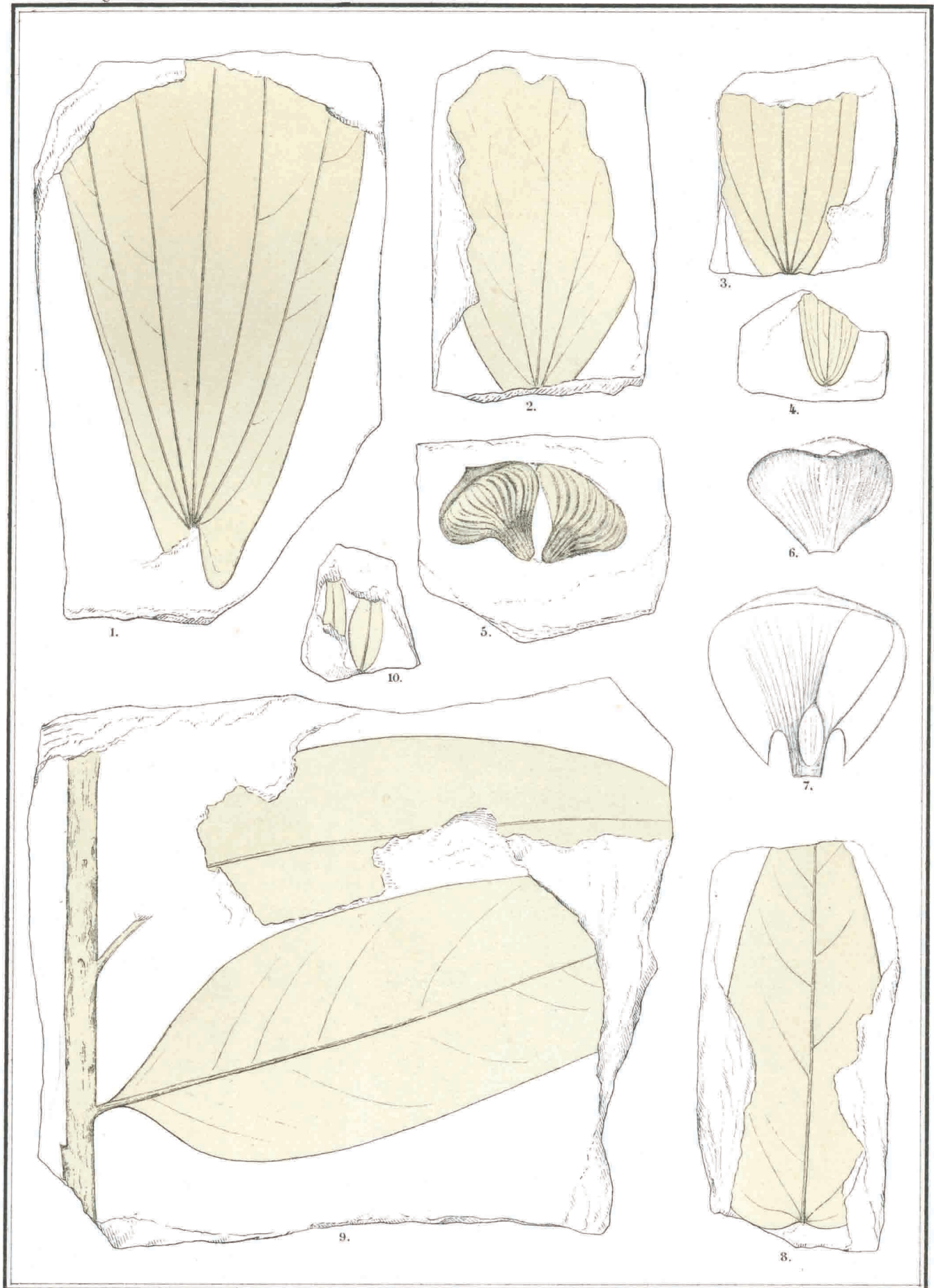
Fig 1. Macclintockia appendiculata . 2-4. M. cretacea . 5. Dammara borealis . 6. D. australis . 7. D. robusta . 8. Ficus Hellandiana . 9. Laurus Odini . 10. Leguminosites Dalageri .
