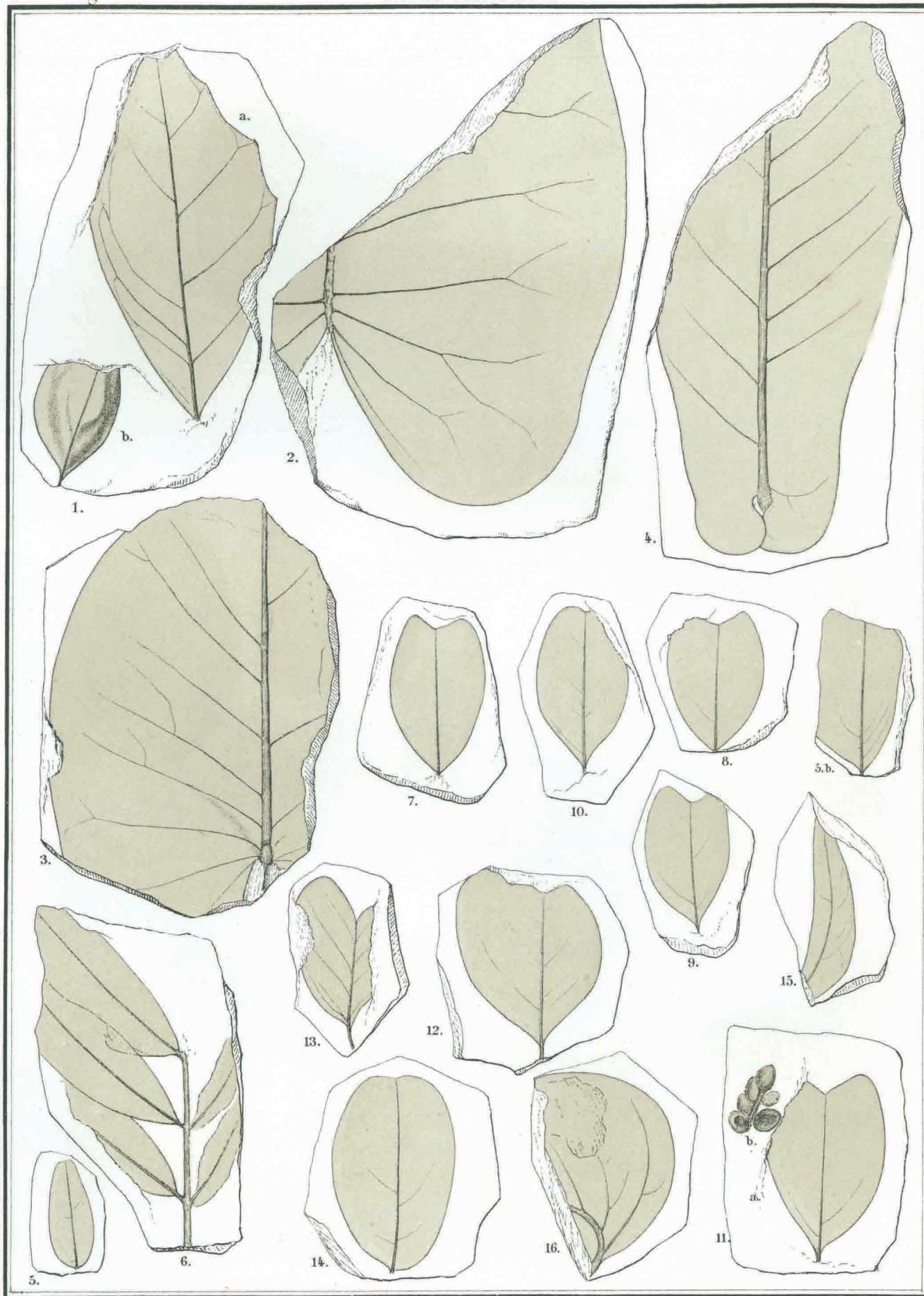
Fig. 1.a. Ilex antiqua . 1.b. Myrsine borealis . 2. 3. Pterospermites cordifolius . 4. Pt. auriculatus . 5. Cassia antiquorum . 6. C. angusta . 7-11. Colutea primordialis . 12. 13. C. valde-inaequalis . 14. Leguminosites ovalifolius . 15. L. macilentus . 16. Phyllites incurvatus .
