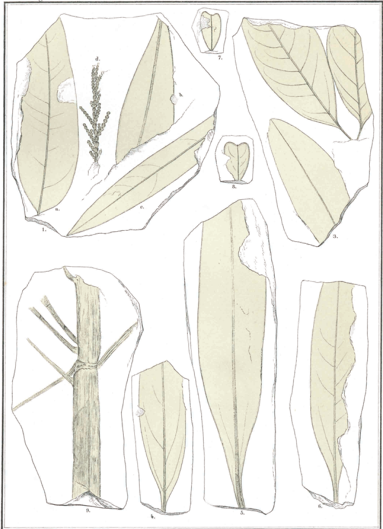
Fig: 1. a, b. Sapindus Morisoni Lesq. 1. c. Laurus angusta . 1. d. Libocedrus cretacea . 3. Juglans arctica . 4.-6. Ficus crassipes . 7. 8. Colutea primordialis . 9. Equisetum amissum .
