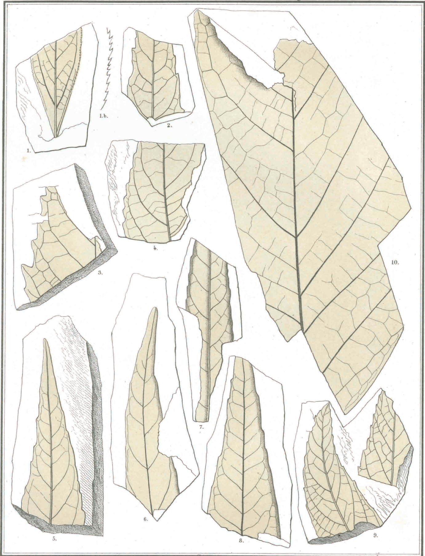
Fig. 1. Ceanothus denticulatus . 2-9. Juglans Heerii Eu. 10. Magnolia Nordenskiöldi .
