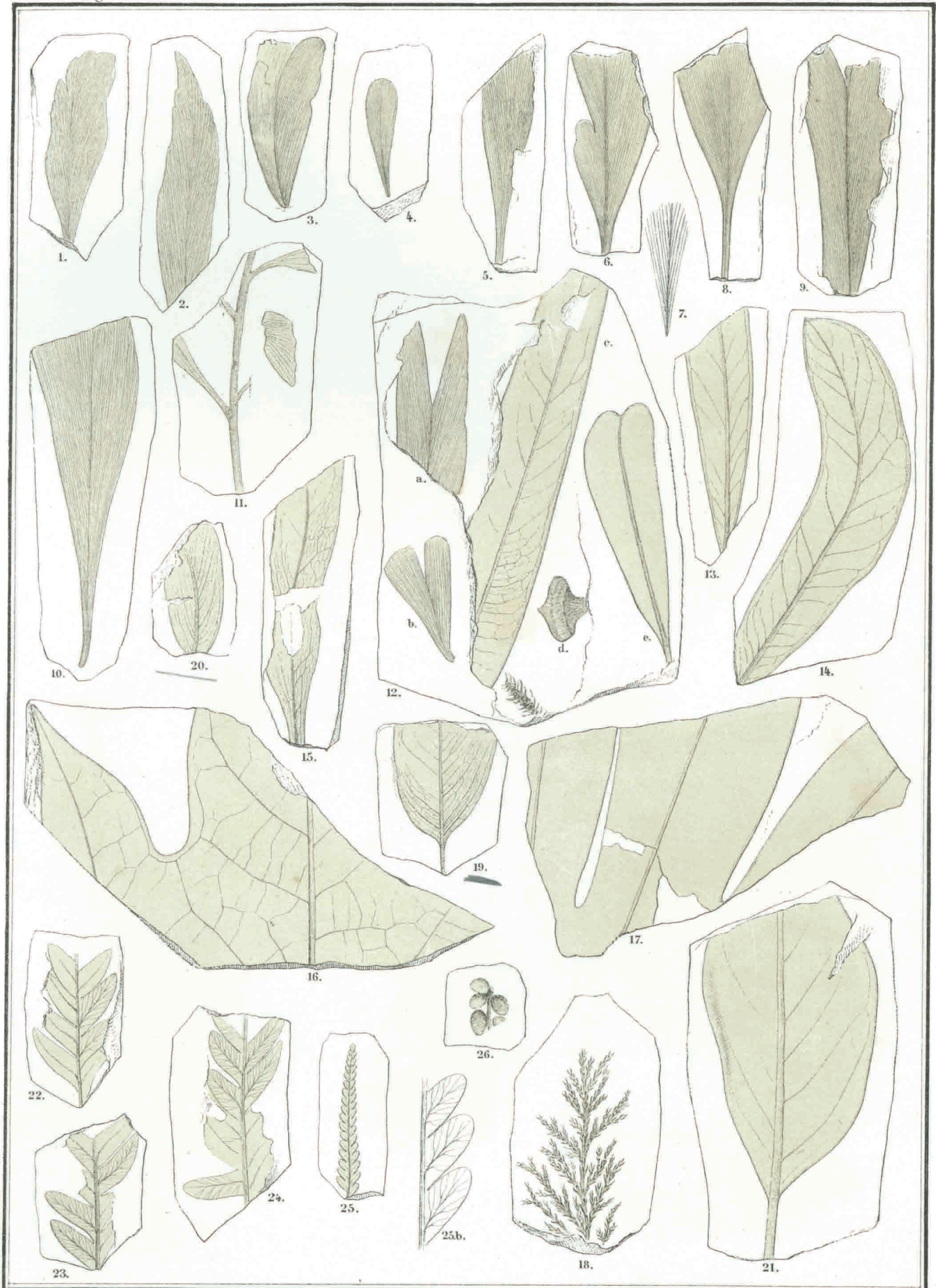
Fig. 1-12. Thinfeldia Lesquereuxiana . 12.c.d. 13. Eucalyptus Geinitzi . 12.e. Myrica emarginata . 14. Eucalyptus borealis . 15. Ficus crassipes . 16. 17. Aralia grönlandica . 18. Juniperus hypnoides . 19. 20. Myrsine borealis . 21. Magnolia alternans . 22-24. Pteris Albertsii Dkr. sp. 25. Gleichenia comptoniaefolia Ett. 26. Myrica .
