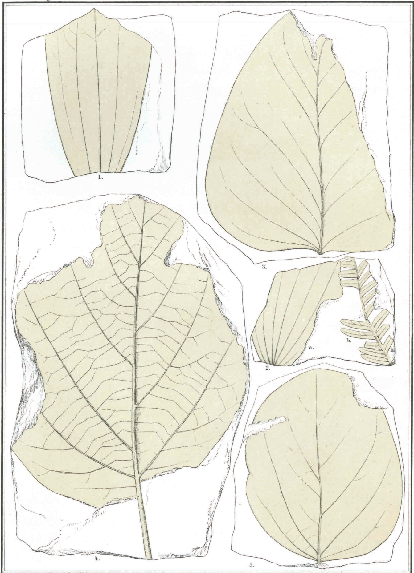
Fig. 1. 2. a. Macclintockia cretacea. 2. b. Pecopteris bohemica. 3. Magnolia Isbergiana. 4. Credneria integerrima Zenk. 5. Apeibopsis Thomseniana.
