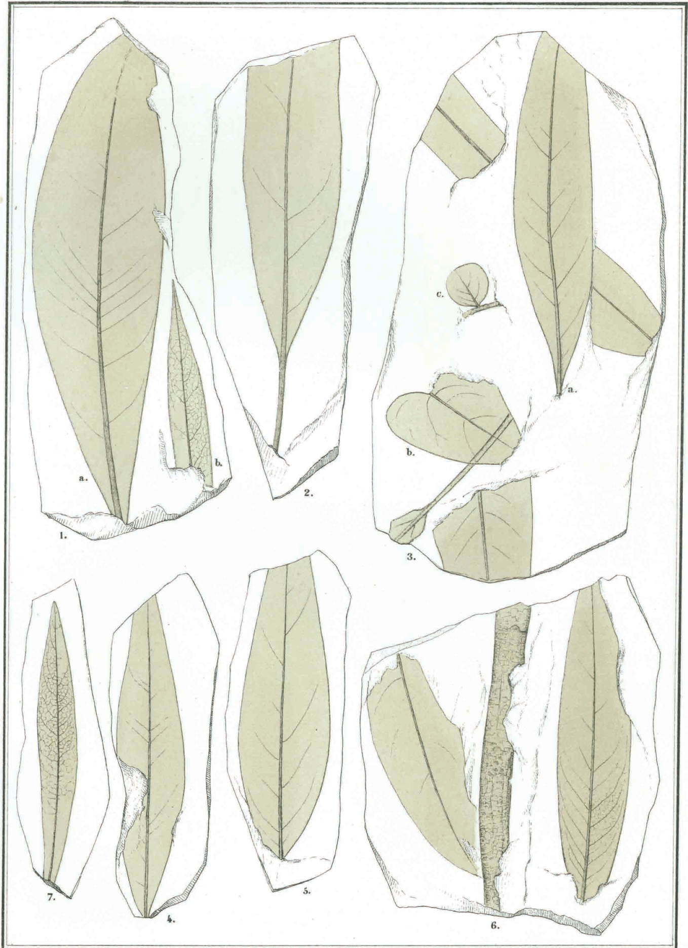
Fig. 1. 2. Ficus atavina . 3. a. 4-6. Laurus plutionia . 1. b. 7. L. angusta . 3. c. Leguminosites orbiculatus .
