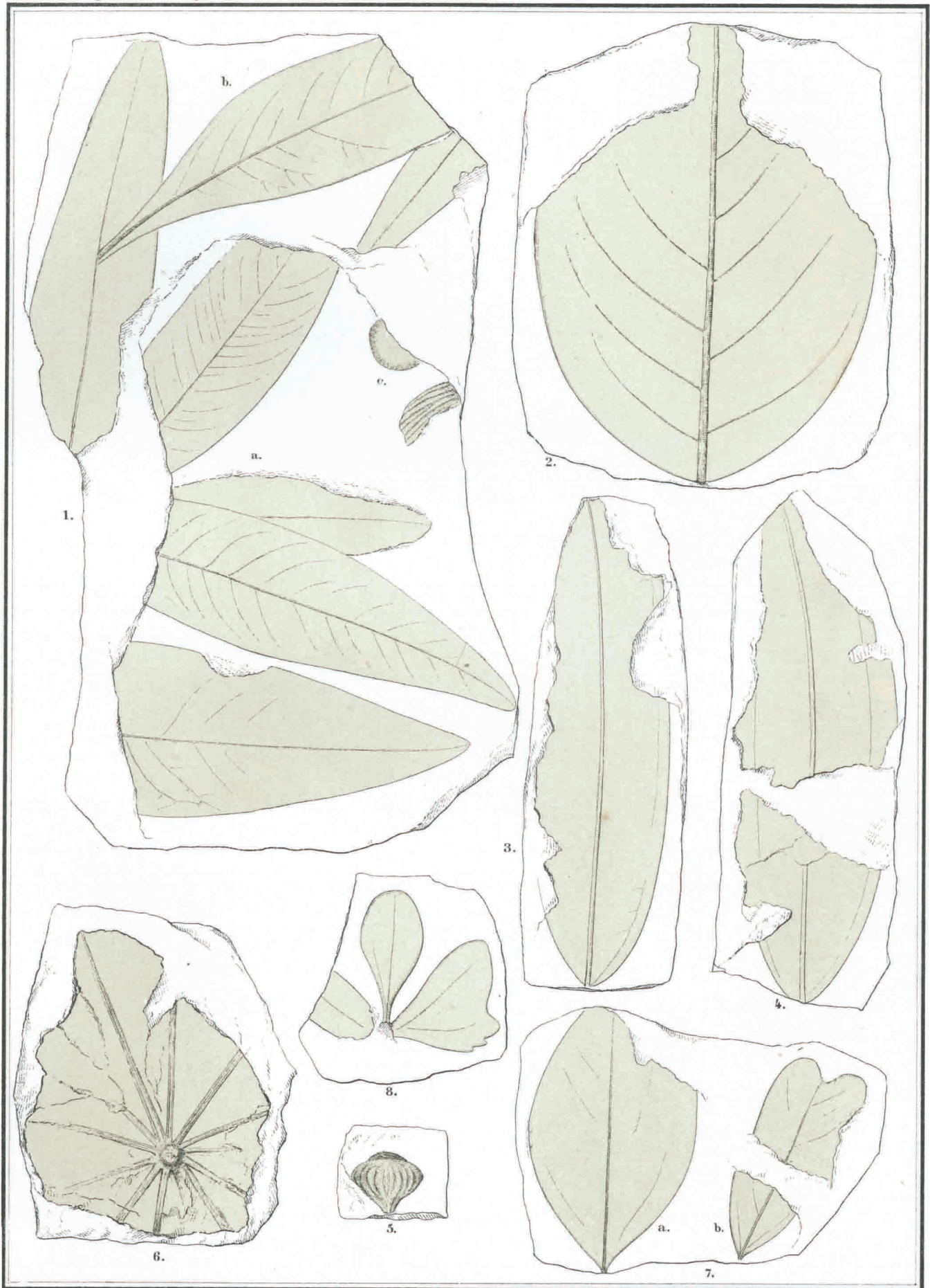
Fig. 1. Sapindus Morisoni Lesq. 2. Juglans arctica . 3. 4. Eucalyptus borealis . 5. Dammara microlepis . 6. Nelumbium arcticum . 7. a. Populus Berggreni . 7. b. Colutea Langeana . 8. Anacardites amissus .
