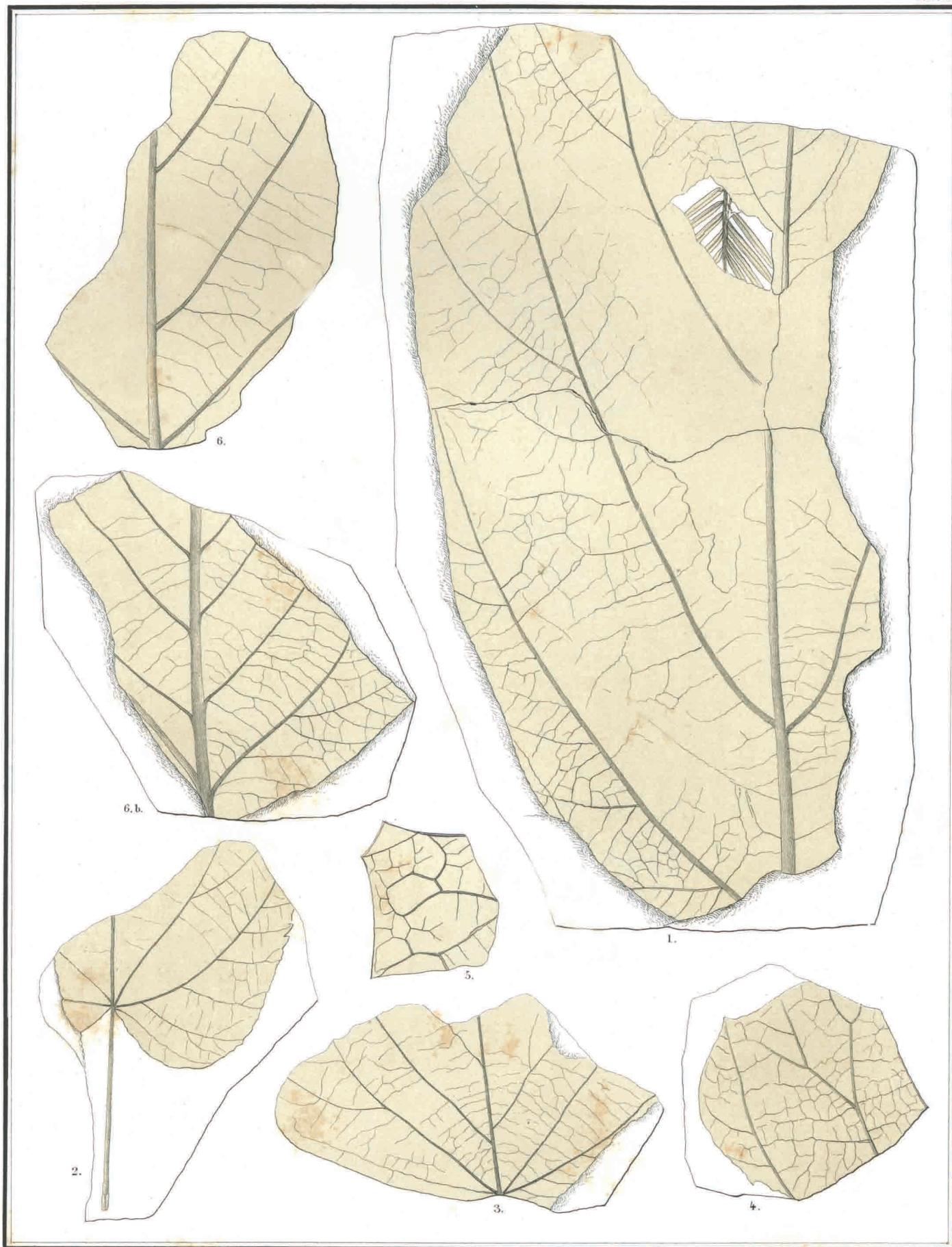
Fig. 1. Magnolia Nordenskiöldi . 2, 3. Tilia Malmgreni . 4, 5. Hedera M'Clurii . 6. Platanus aceroides .
