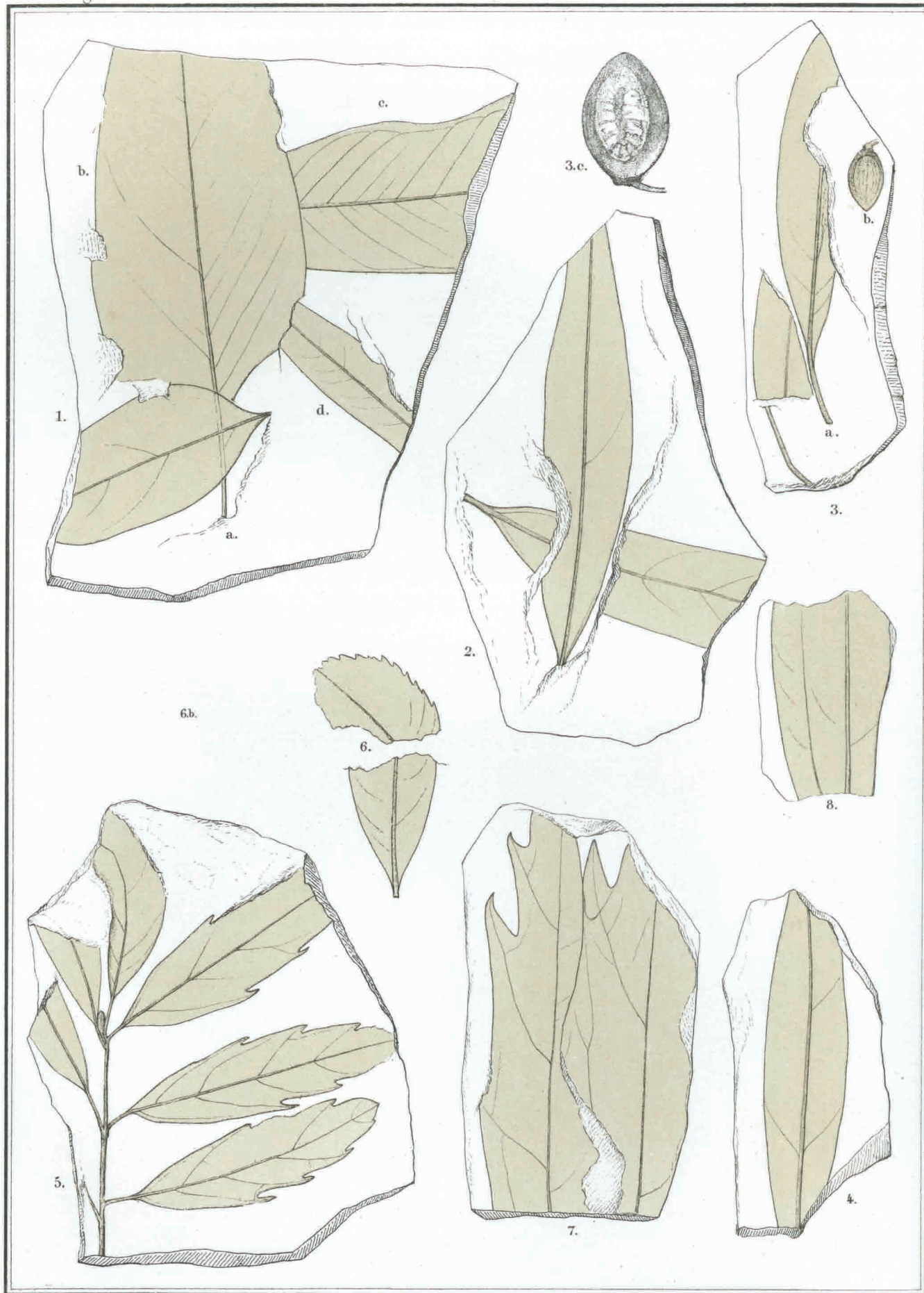
Fig: 1.a. Populus Berggreni. 1.b. Ficus atavina. 1.c. Eucalyptus Geinitzi. 1.d. 2.3.4. Laurus plutonia. 5. Quercus Rinkiana. 6. Q. Warmingi. 7. Q. ferox. 8. Cinnamomum sezannense Wal.
