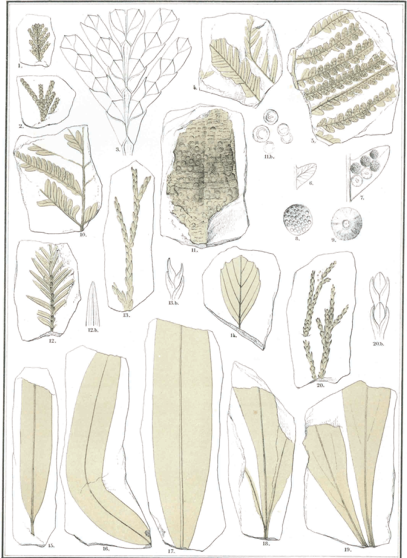
Fig. 1-3. Libocedrus cretacea . 4. Aspidium Jensenii . 5-9. A. fecundum . 10. Dicksonia conferta . 11. Xylomites aggregatus . 12. Cuninghamites borealis . 13. Cyparissidium gracile . 14. Quercus troglodites . 15-17. Myrica longa . 18. 19. Dewalquea grönlandica . 20. Thuites Meriani .
