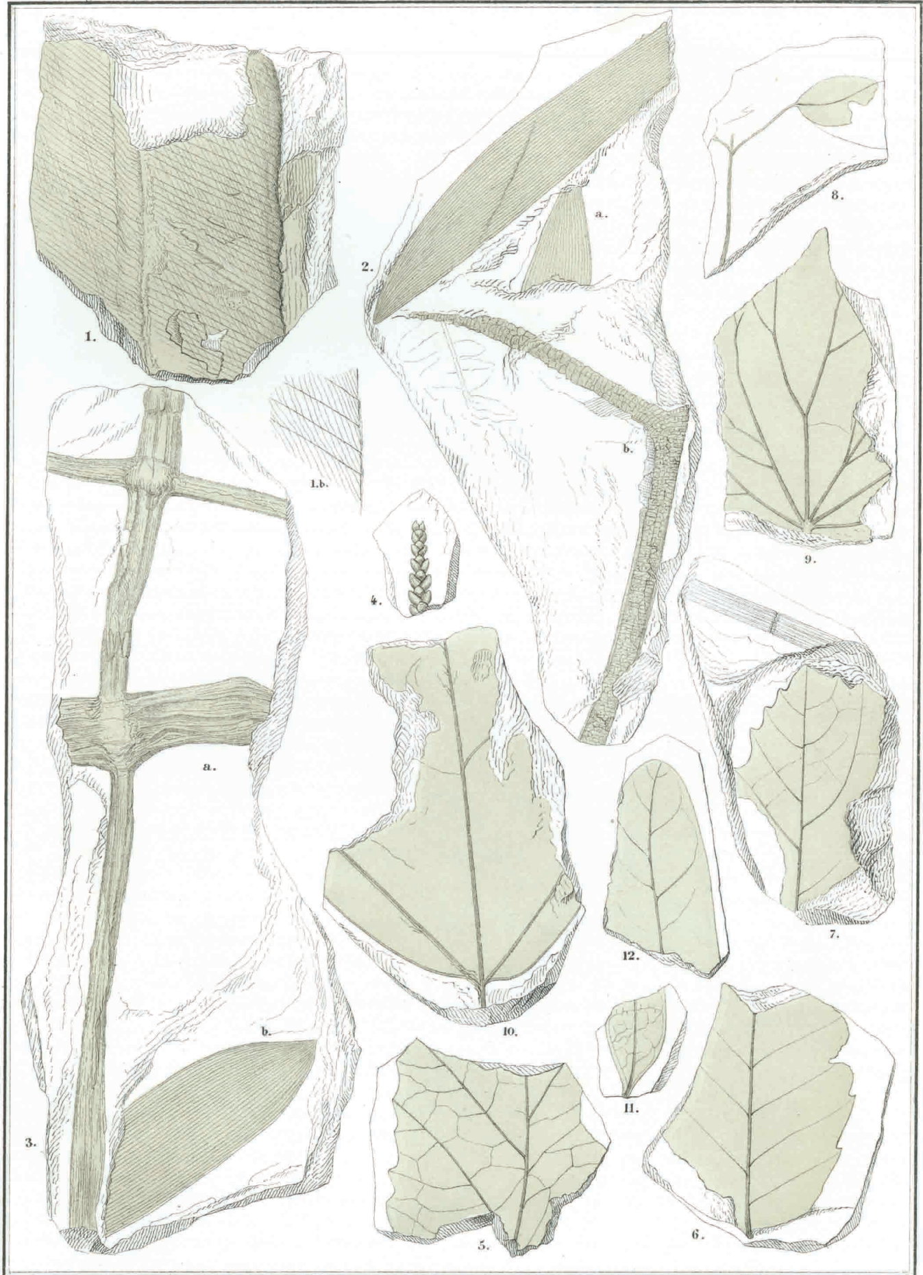
Fig. 1. Alisma? reticulata . 2. a. 3. b. Podozamites latipennis . 3. a. Equisetum amissum . 4. Thuides . 5. 6. 7. Quercus westfaliae fls. 8. Phyllites longepetiolatus . 9. 10. Hedera primordialis Sap. 11. Myrtophyllum parvulum . 12. Magnolia obtusata .
