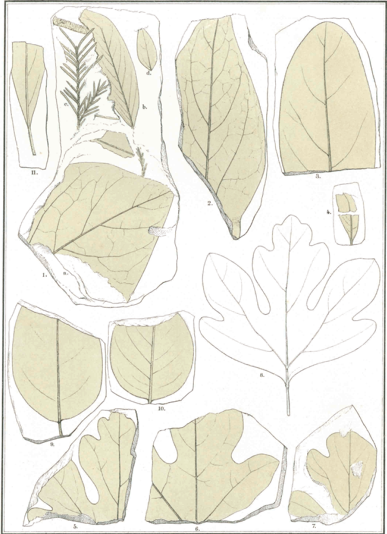
Fig. 1.a. Populus . 1.b. II Andromeda Parlatorii . 1.c. Sequoia rigida . 2. Magnolia alternans . 3. Magnolia obtusata . 4. Myrtophyllum parvulum . 5-8. Cissites formosus . 9. 10. Rhamnus Oerstedii .
