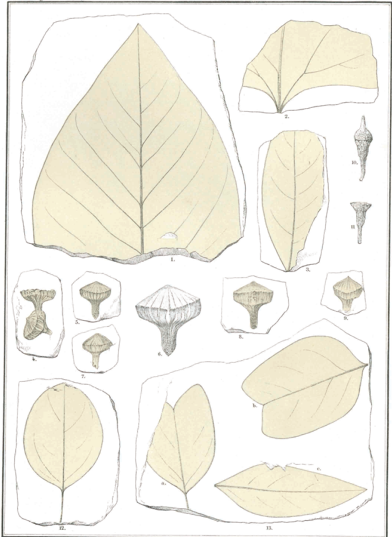
Fig. 1. Magnolia Capellinii . 2. Hedera cuneata . 3. Laurus Hollae . 4-9. Eucalyptus Geinitzi . 10. 11. F. robusta Sm. 12. Populus Berggrenii . 13. a. b. Liriodendron Meekii . 13. c. Rhamnus acuta .
