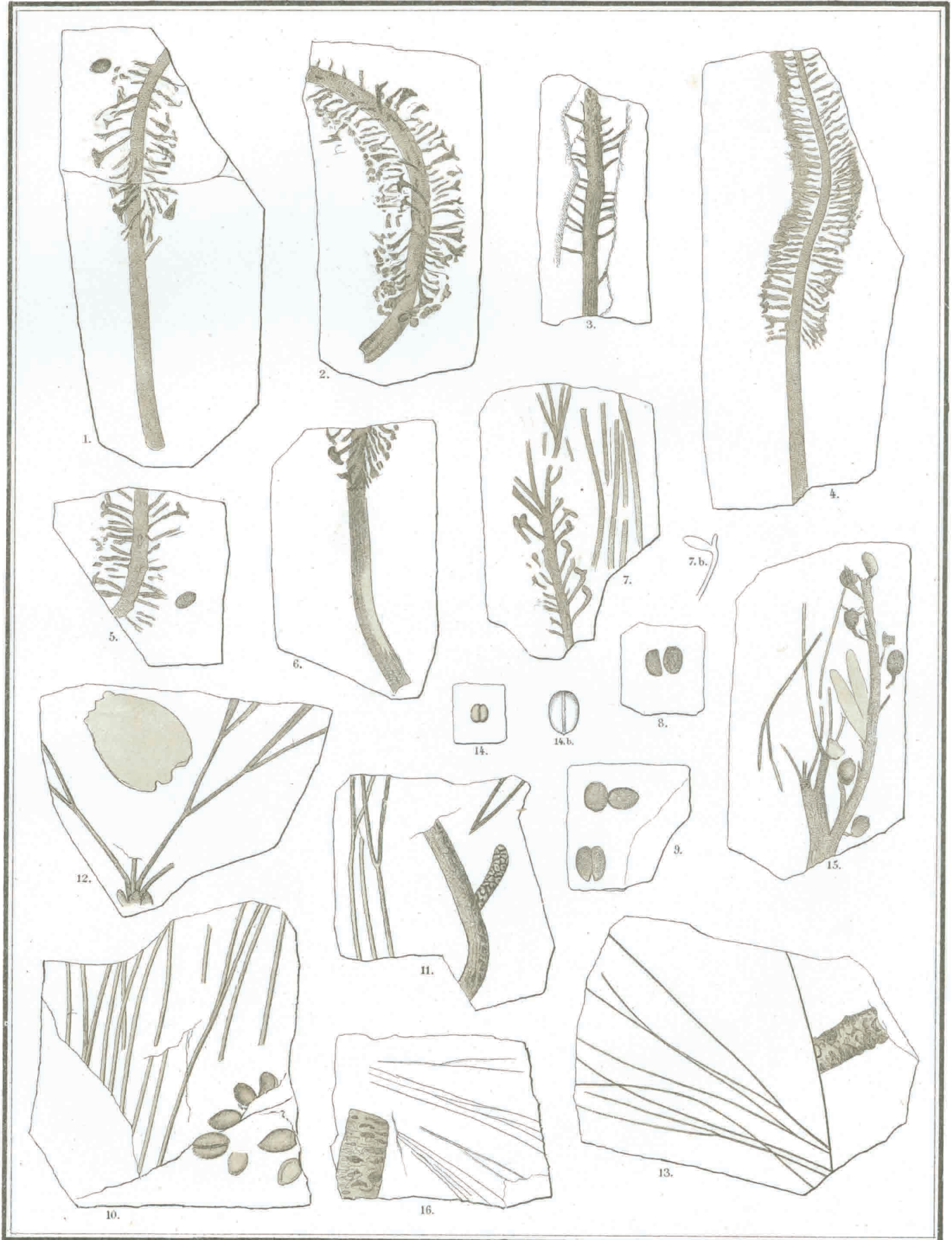
Fig. 1-6. Ginkgo grandiflora . 7-12. Czekanowskia rigida . 13-16. C. setacea .
