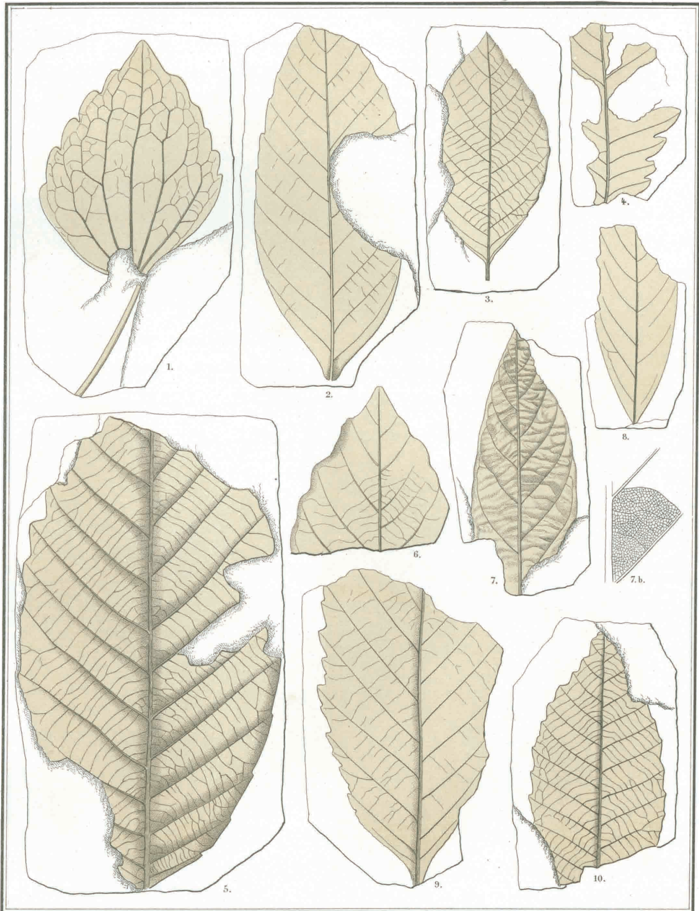
Fig. 1. Populus arctica . 2, 3. Fagus Deucalionis . 4. Quercus pseudocastanea . 5. Q. grönlandica . 6-8. Q. Lyelli . 9. Q. Olafseni . 10. Castanea Ungeri .
