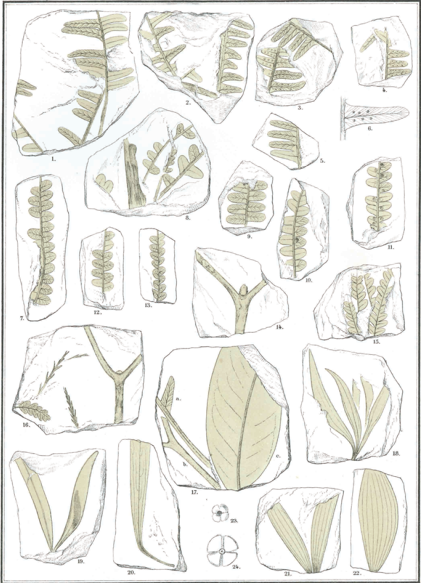
Fig 1-6. Aspidium Jenseni . 7.-14. 15. 16. Gleichenia obtusata . 17. a. Pteris frigida . 17. c. Laurus Hollae . 18. Baiera sagittata . 19. 20. Acerates arctica . 21. Majanthemophyllum lanceolatum . 22. M. cretaceum . 23. Celastrus .
