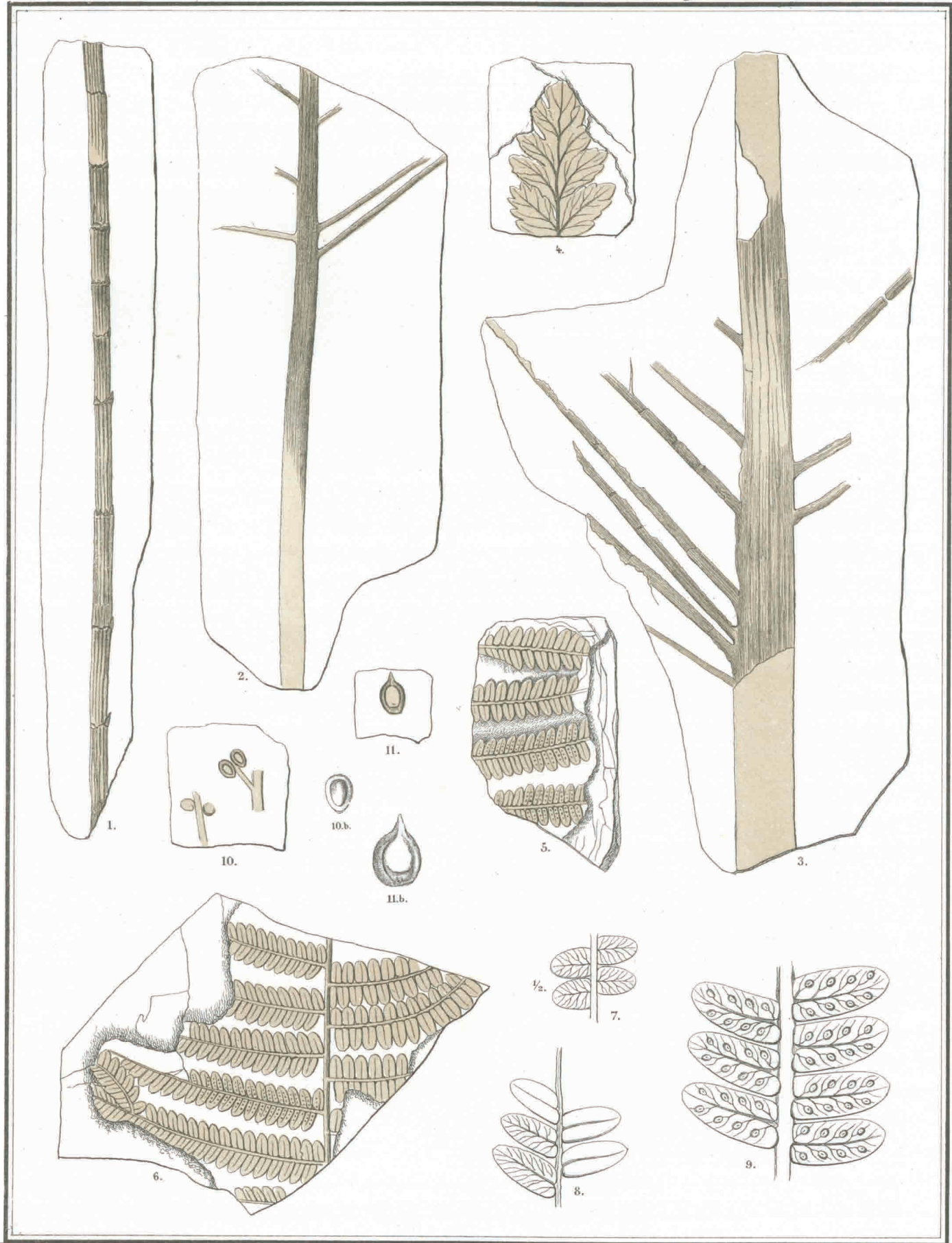
Fig 1-3. Frenelopsis Hoheneggeri . 4. Pecopteris Bolbroeana . 5-9. P. Andersoniana .
