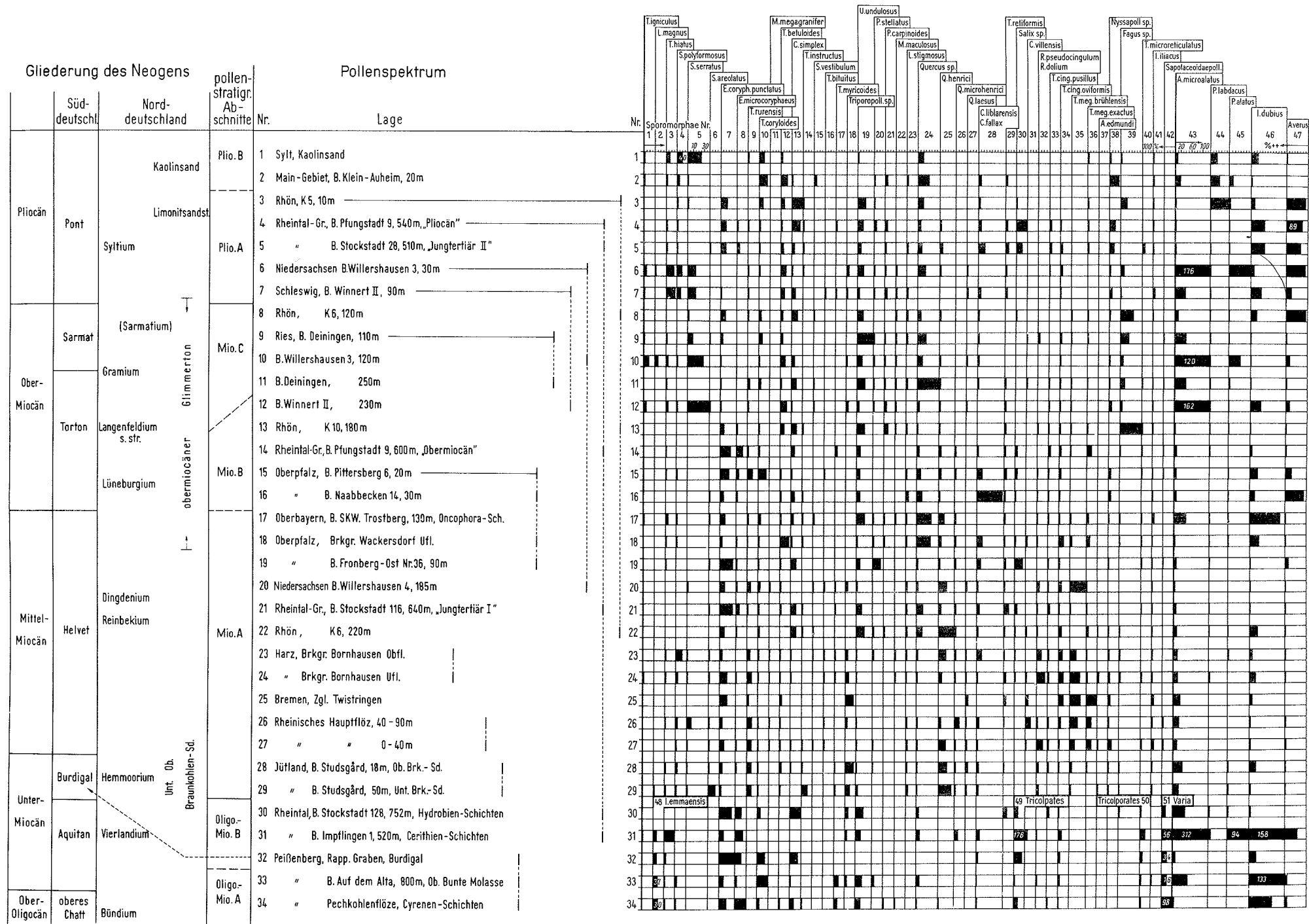
Abb. 2 Pollenstratigraphische Gliederung des Miozäns in Mitteleuropa auf Grund von Durchschnittsspektren in besonderer Darstellung.
