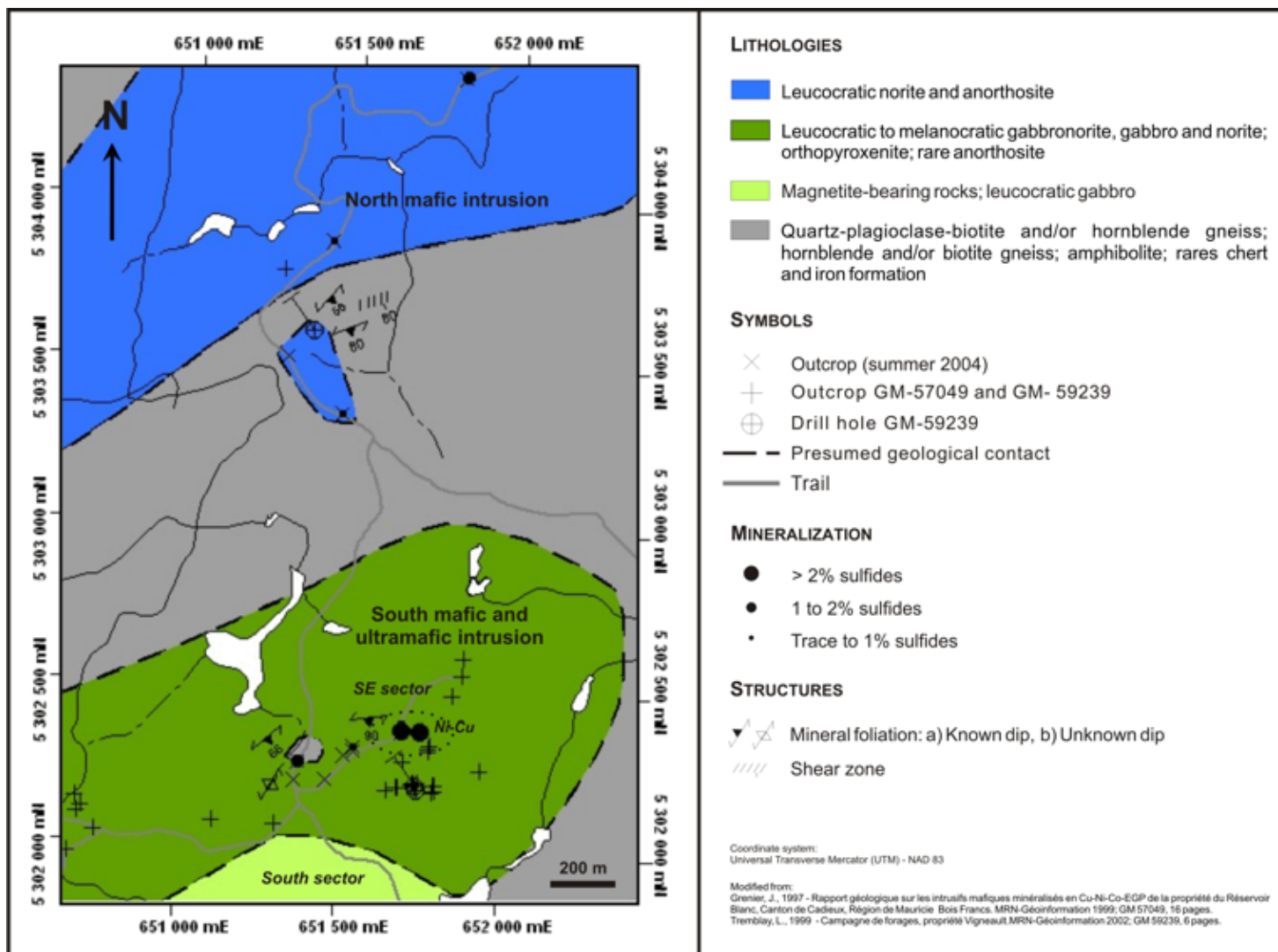
FIG. S1 Geology of the Réservoir Blanc prospect area
