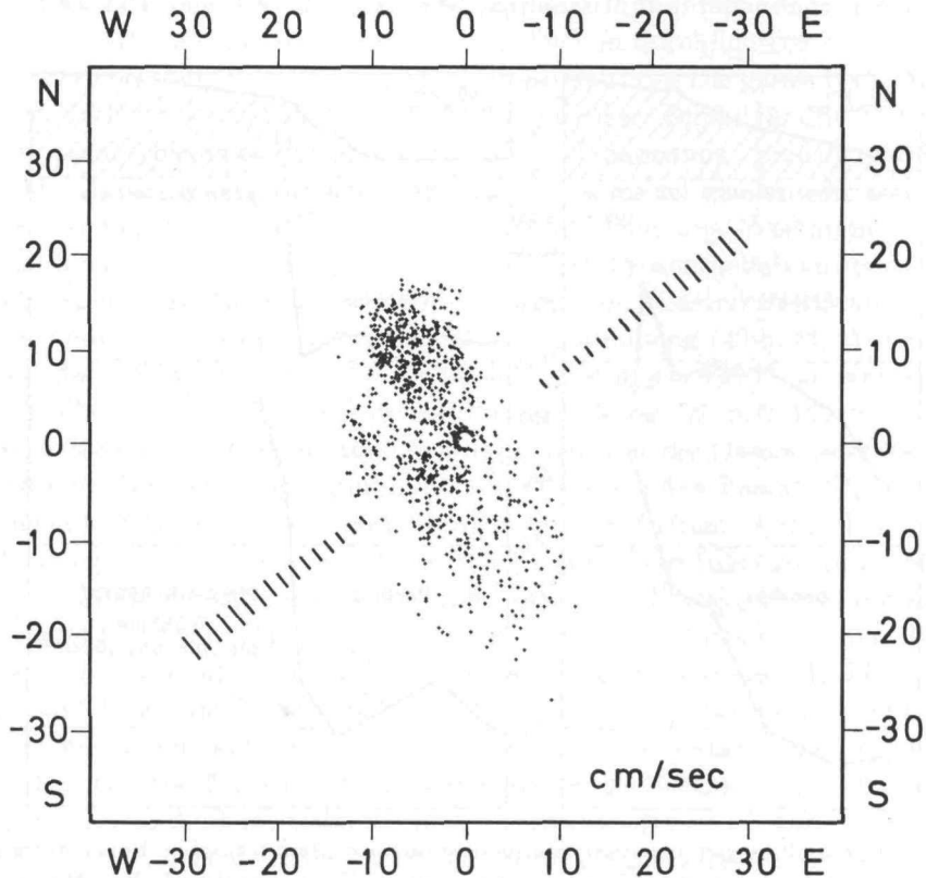
Abb. 3. Vektorverteilung von Strömungen vor Marokko in 175 m Wassertiefe, 5 m über dem Meeresboden. Verlauf des Schelfrands gestrichelt. Nach SIEDLER & SEIBOLD (1973).
