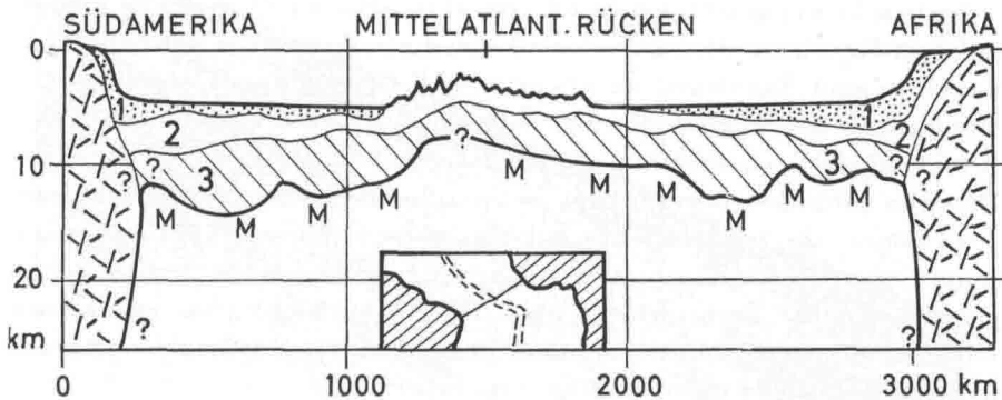
Abb. 13. Profil durch den äquatorialen Atlantischen Ozean. Lagenhafter Aufbau des ozeanischen Untergrunds nach refraktionsseismischen Untersuchungen. Lage 1 = Sedimente, Lage 2 = Übergangslage mit meist rauher Oberfläche aus Basaltergüssen, Lage 3 = ozeanische Kruste aus basischen Tiefengesteinen, M = oberer Mantel. Art des Übergangs zur kontinentalen Kruste noch unklar. Vereinfacht nach
