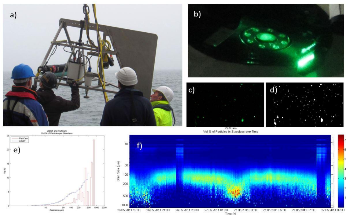
Abbildung 11: MARUM Partikelkamera "PCAM II" (G. Herbst & C. Winter) a) Einsatz in Tidegewässern im Messrahmen: PCAM II mit Sequoia LISST100X, ECM-CTD an Bord FS Heincke; b) Messvolumen im Laserfeld, c) Originalbild Partikel, d) optimiertes Binärbild Partikel, e) berechnete Partikelgrößenverteilung durch Bildanalyseverfahren, f) Zeitreihe der berechneten Partikelverteilung für einen Tidezyklus.
