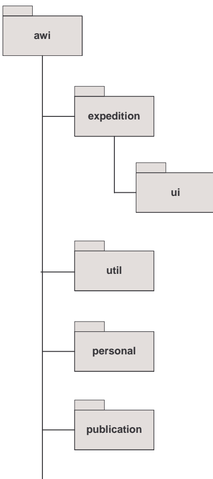
Abbildung 33: Paketstruktur
